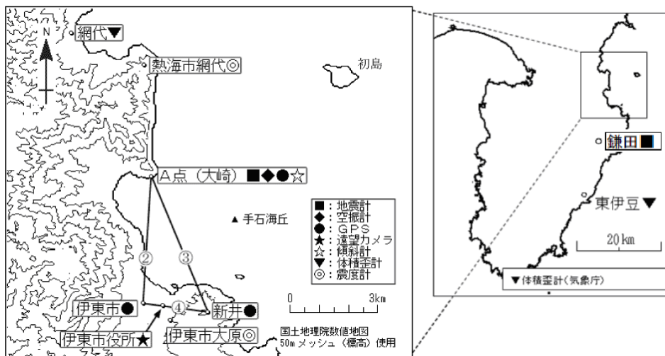
図3 伊豆東部火山群 気象庁の観測点配置図(小さな白丸は観測点位置を示しています) GPS基線 ~ は図2の ~ に対応しています。
