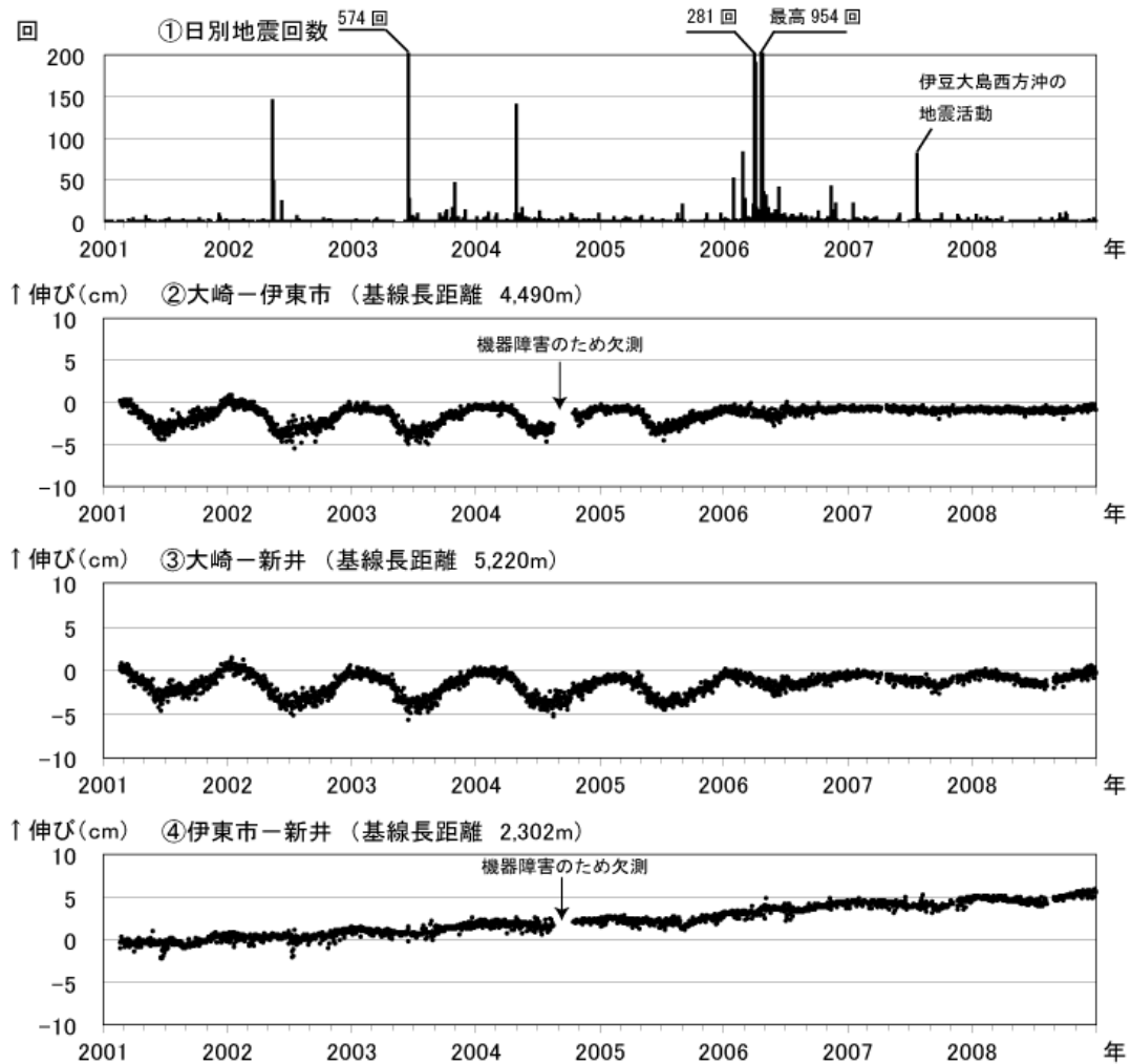
図2 伊豆東部火山群 最近の火山活動の推移（2001年1月～2009年1月）
