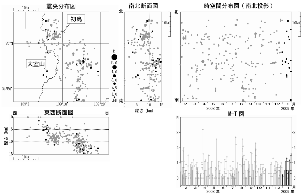
図 1※ 伊豆東部火山群 震源分布図（2008 年 2 月 1 日～2009 年 1 月 31 日）
