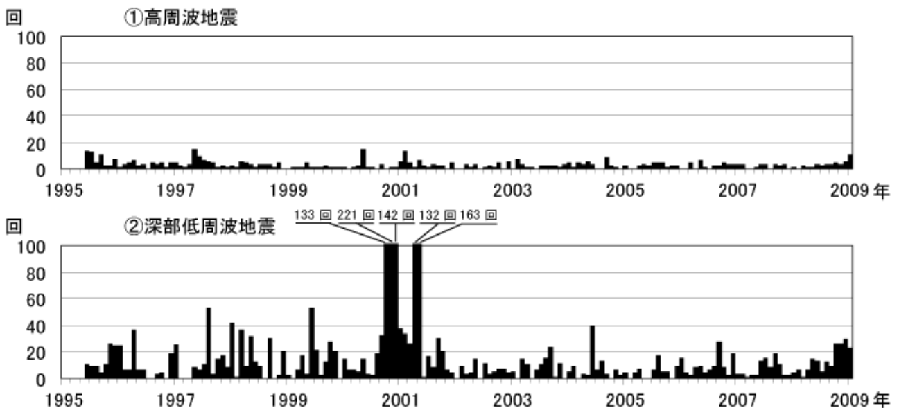
図 1 富士山 月別地震回数(1995 年 6 月～2009 年 1 月)
