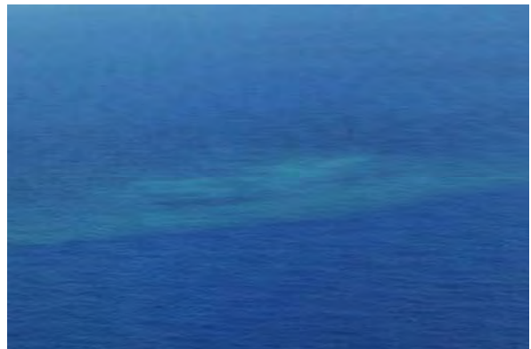
図 2※ 福德岡ノ場 変色水の状況 （11 日、北側から撮影）
