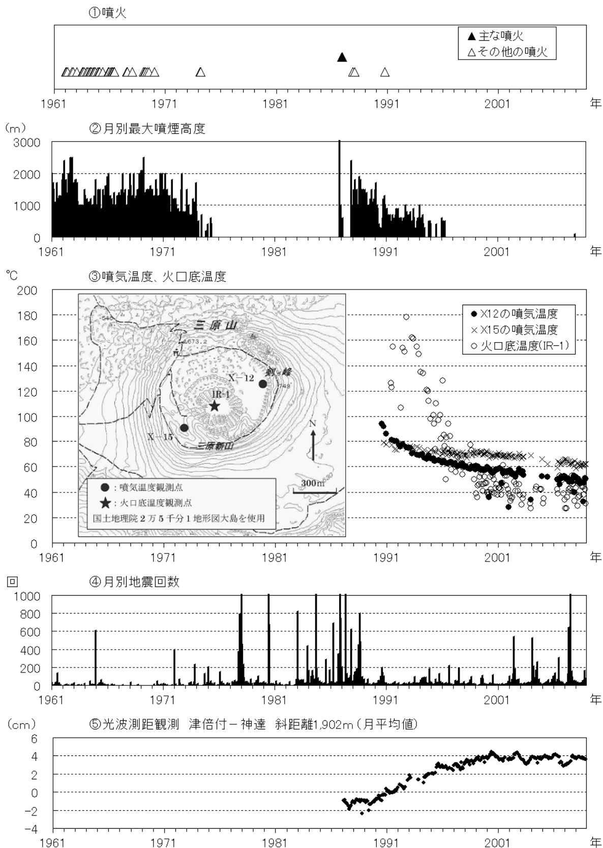
図4 伊豆大島 長期間の火山活動経過図（1961年1月～2008年11月）
