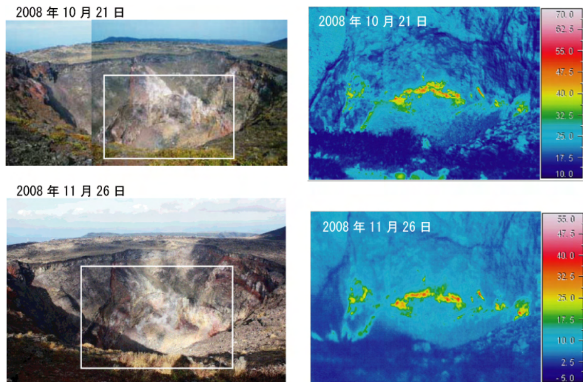
図 2 伊豆大島 中央火口北側内壁の状況（左）と地表面温度分布 1) （右） （左の写真の白枠部分が右の赤外熱映像撮影部分）
