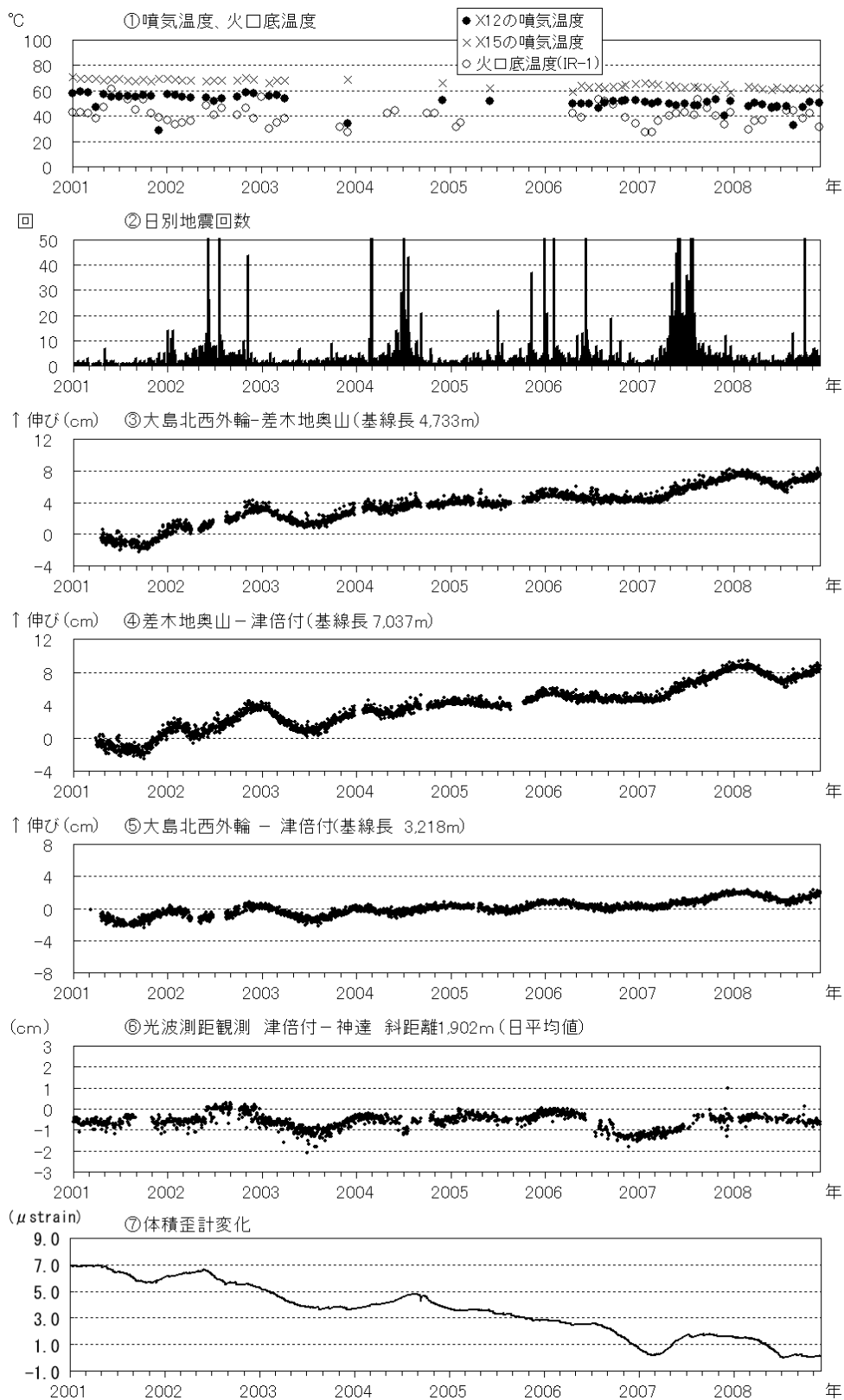
図5 伊豆大島 最近の火山活動経過図（2001 年 1 月～2008 年 11 月）
