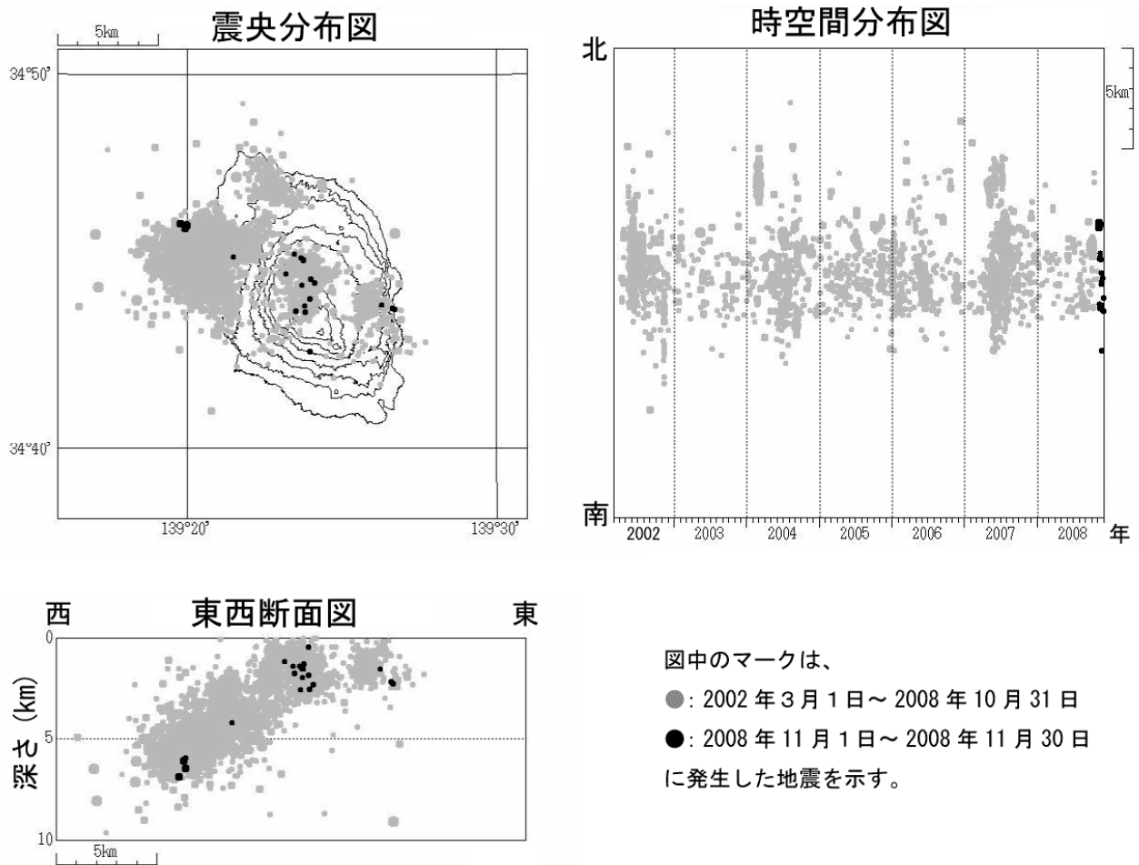
図 6※ 伊豆大島 震源分布図（2002 年 3 月 1 日～2008 年 11 月 30 日）
