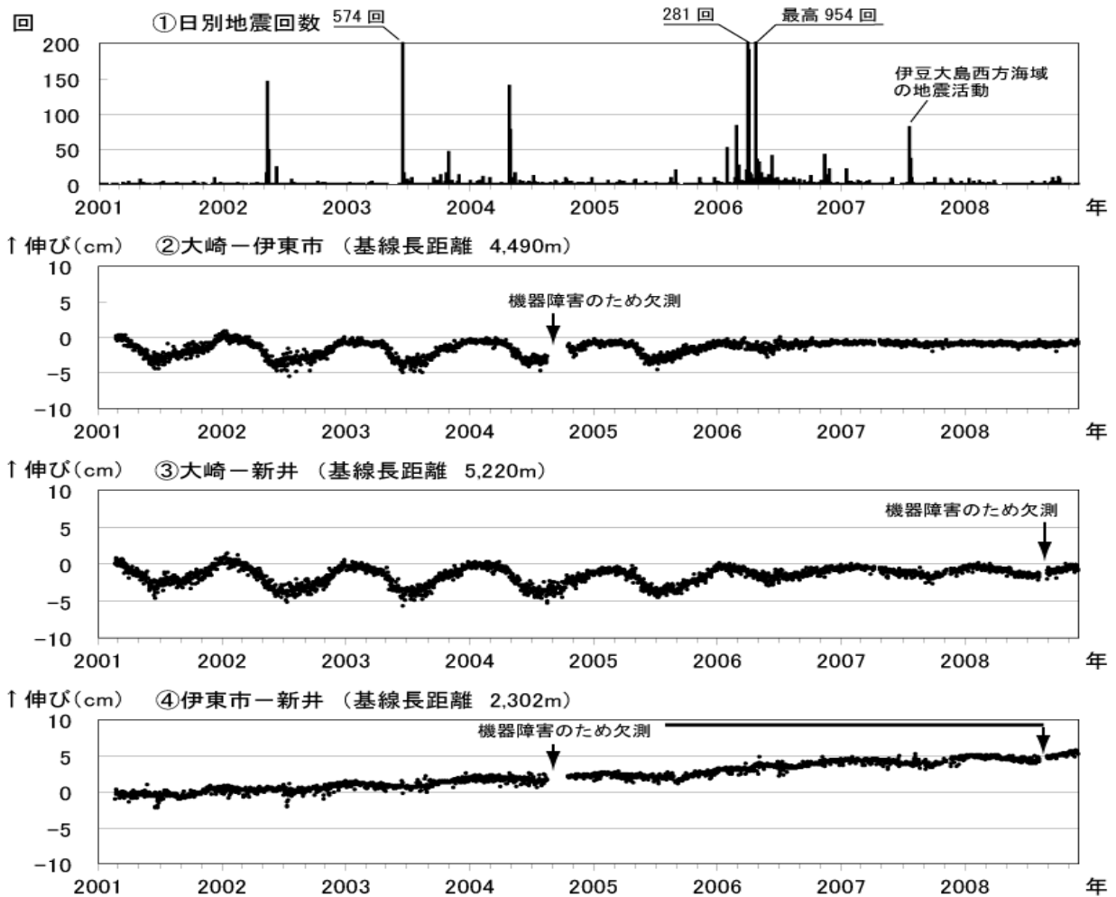
図2 伊豆東部火山群 最近の火山活動の推移 (2001年1月~2008年11月)
