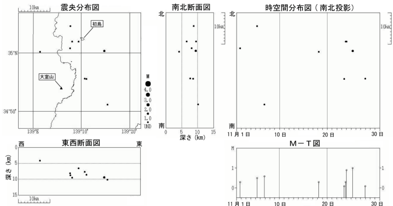
図 1※ 伊豆東部火山群 震源分布図（2008 年 11 月 1 日～30 日）
