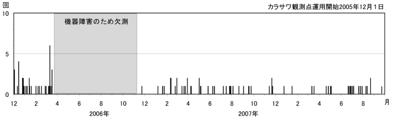
図2 新潟焼山 日別地震回数（2005年12月1日～2008年9月30日）
