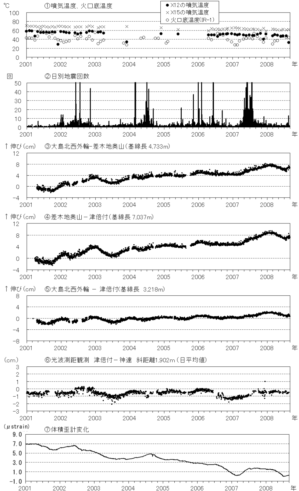
図5 伊豆大島 最近の火山活動経過図（2001年1月～2008年8月）
