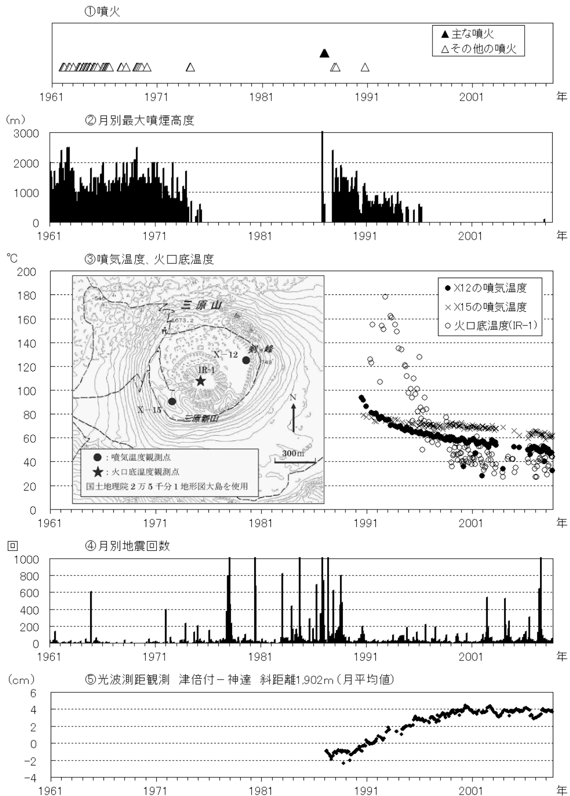
図 4 伊豆大島 長期間の火山活動経過図（1961 年 1 月～2008 年 8 月）
