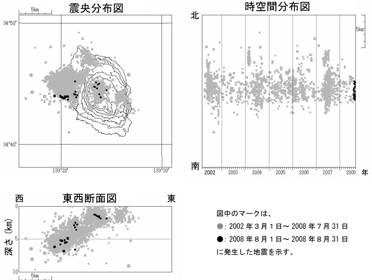
図 6 伊豆大島 震源分布図（2002 年 3 月 1 日～2008 年 8 月 31 日）
