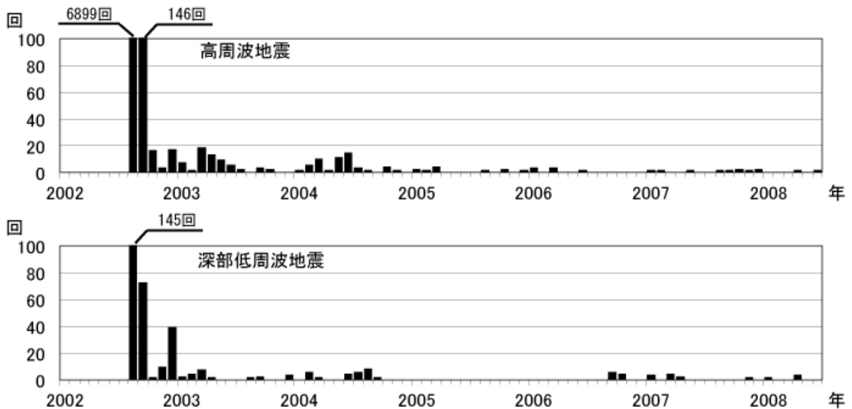
図 1 八丈島 月別地震回数(2002 年 1 月～2008 年 6 月)
