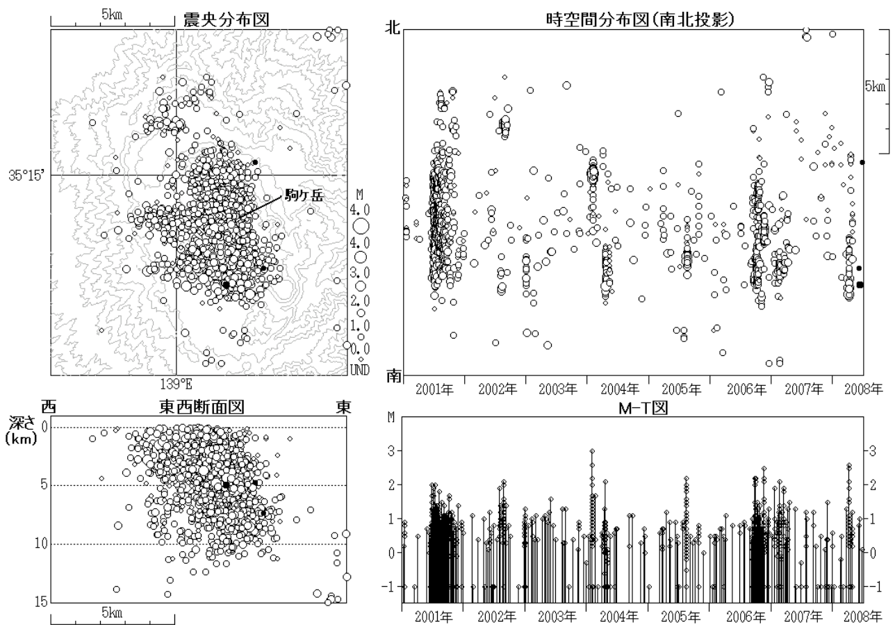
図3 箱根山 地震活動経過(2001年1月1日~2008年6月30日)
