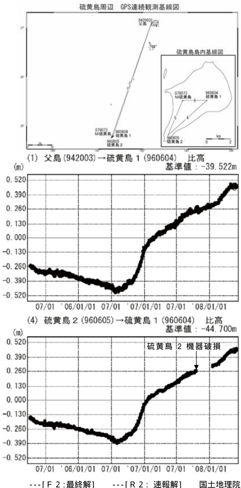
図1 硫黄島 国土地理院によるGPS観測結果 1) 2005年1月1日から2008年5月31日までの硫黄島の動き 上のグラフ: 父島に対する硫黄島1の比高の変化 下のグラフ: 硫黄島2(島南西部の摺鉢山付近)に対する硫黄島1(島北部の元山地域)の比高の変化
