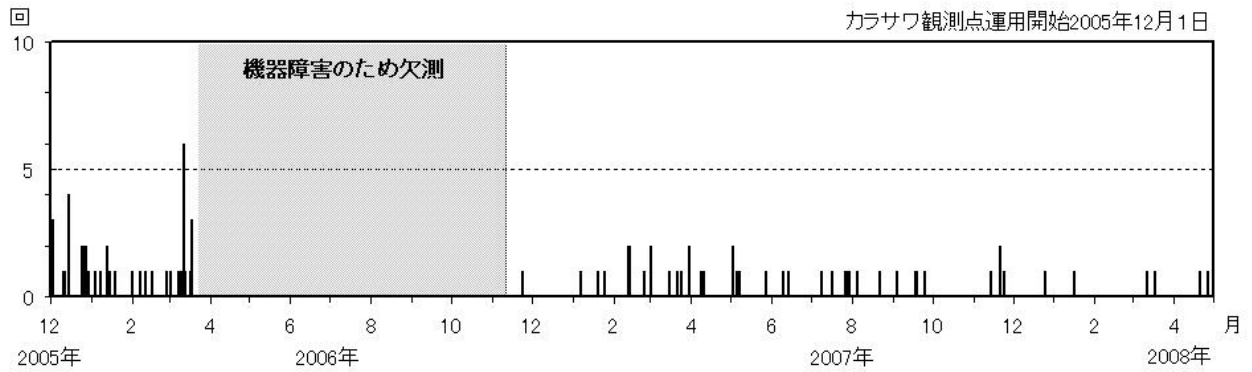
図 2 新潟焼山 日別地震回数（2005 年 12 月 1 日～2008 年 4 月 30 日）
