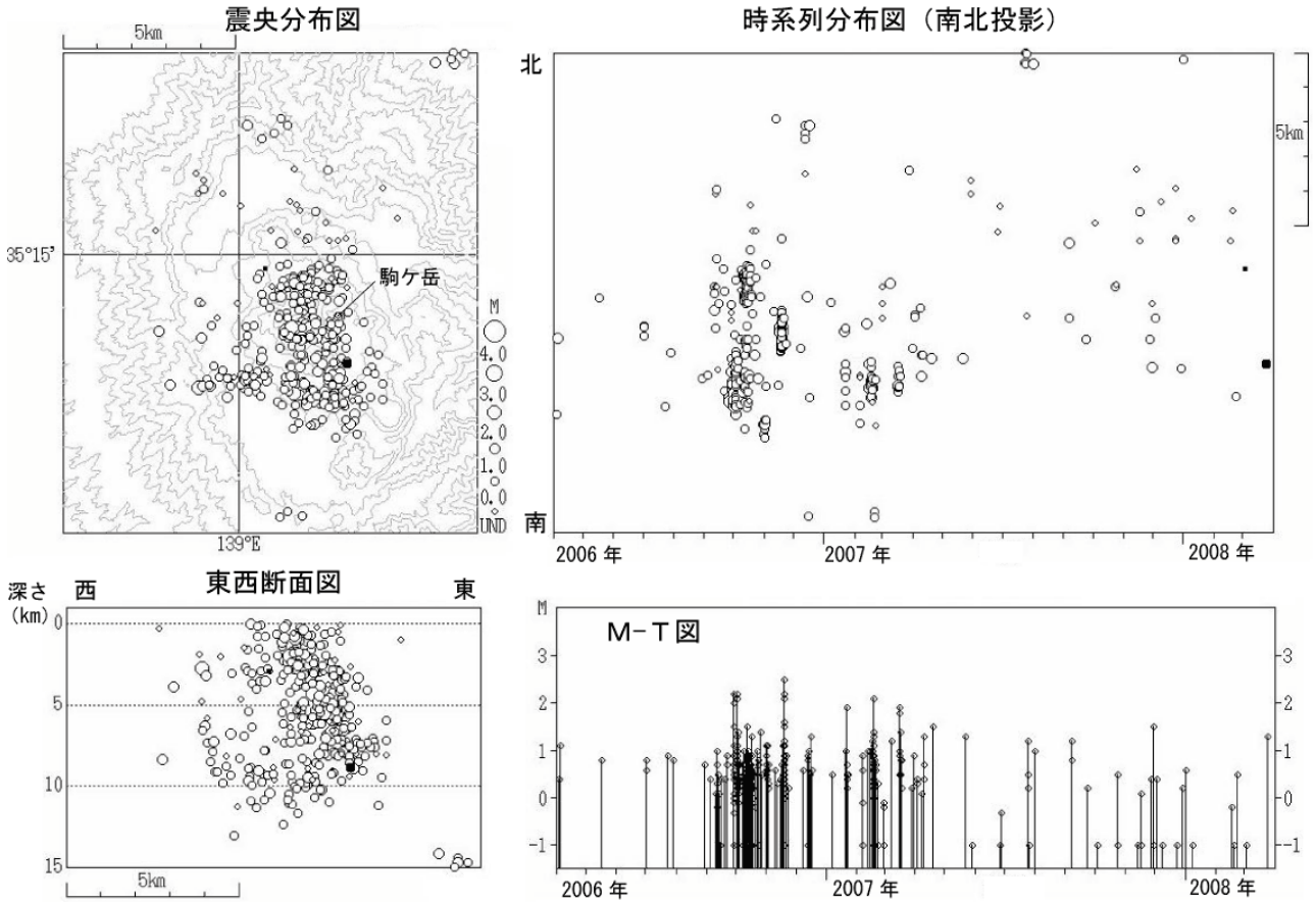
図 2 箱根山 地震活動経過（2006 年 4 月 1 日 ~ 2008 年 3 月 31 日）
