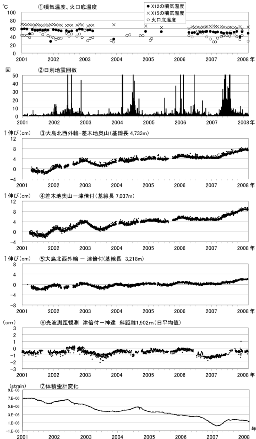
図5 伊豆大島 最近の火山活動経過図(2001年1月~2008年2月)
