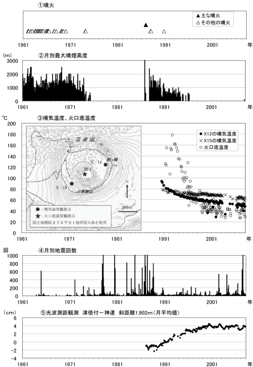
図 4 伊豆大島 長期間の火山活動経過図（1961 年 1 月～2008 年 2 月）
