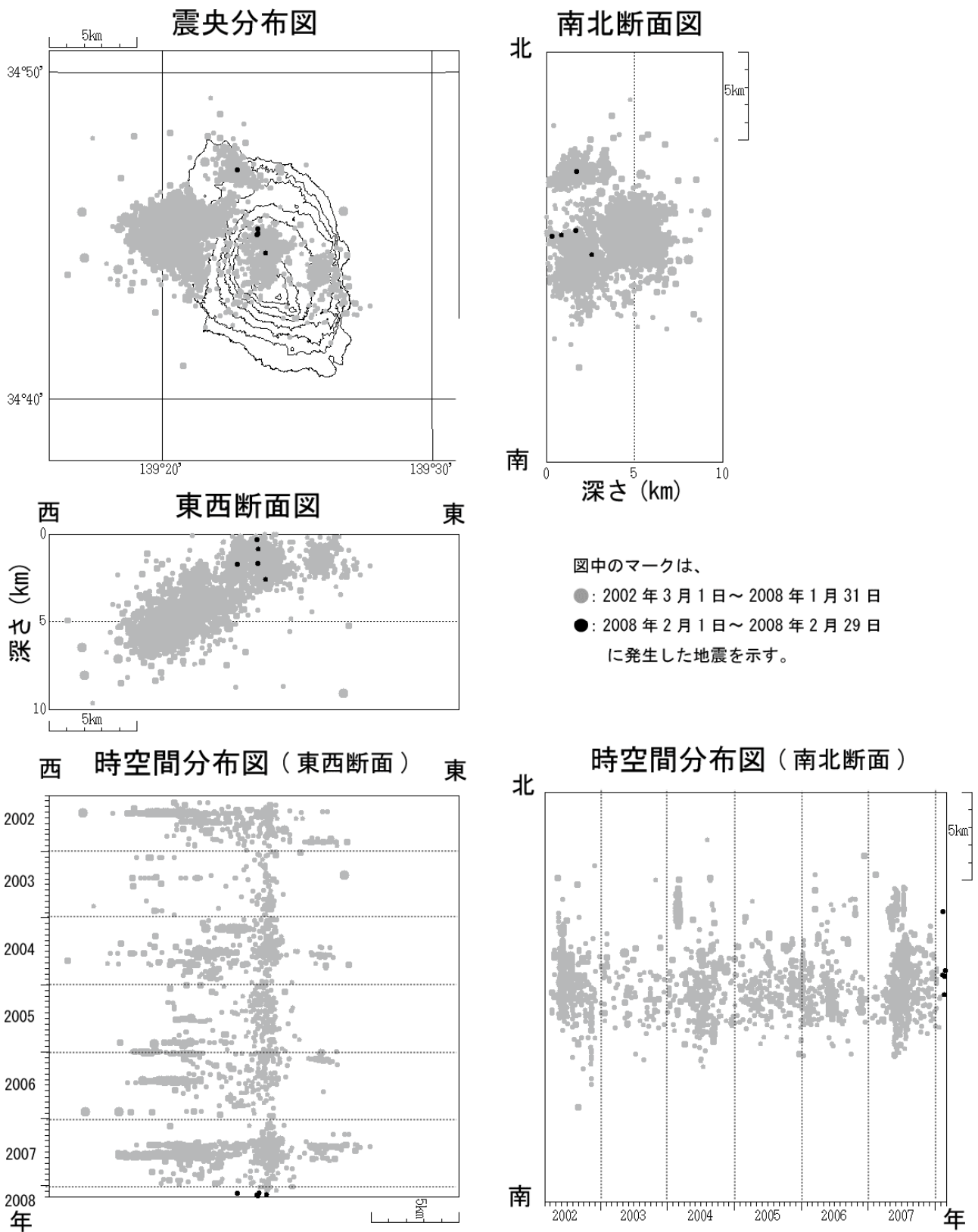
図6 伊豆大島 震源分布図（2002年3月1日～2008年2月29日）
