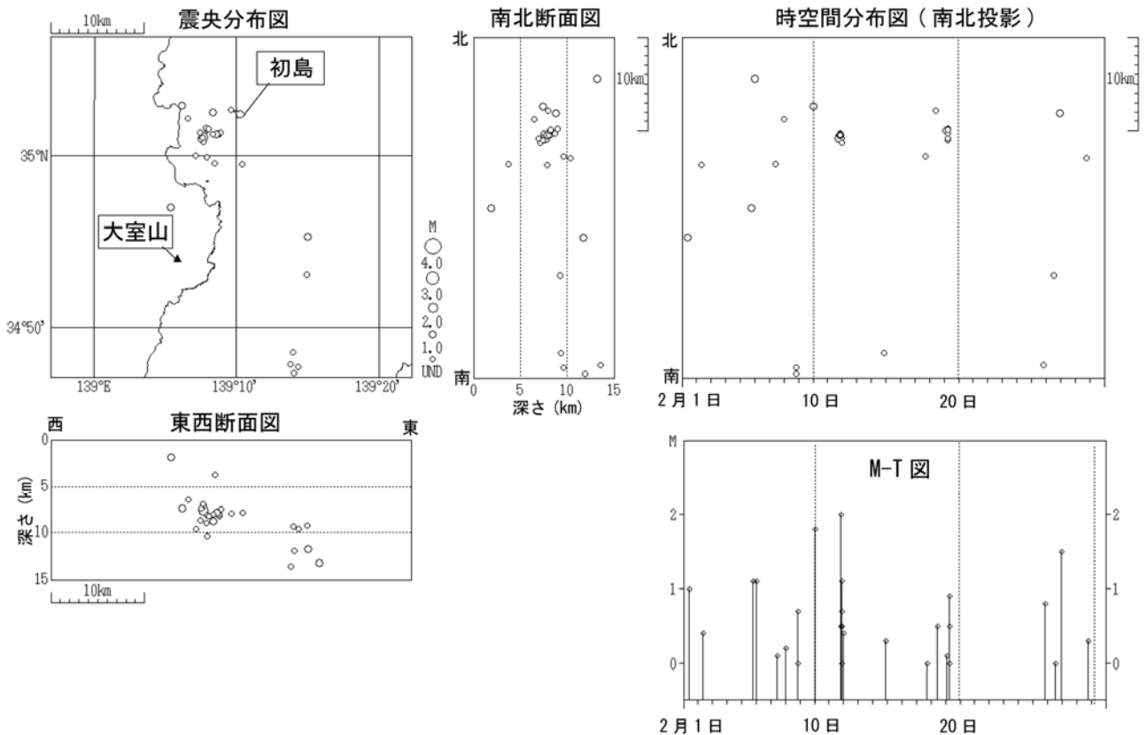
図 1 伊豆東部火山群 地震活動経過図（2008 年 2 月 1 日～ 2 月 29 日）
