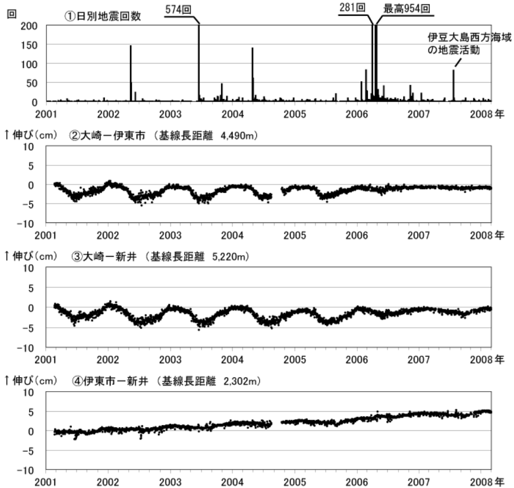
図2 伊豆東部火山群 最近の火山活動の推移（2001年1月～2008年2月） 鎌田地震観測点による日別地震回数 ~ GPS連続観測による基線長変化（観測開始は2001年3月） 基線長変化に見られる冬季の伸びと夏季の縮みの傾向は季節変動による変化です。 ~ は図3のGPS基線 ~ に対応しています。
