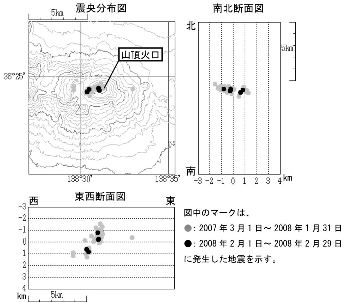
図 3 浅間山 火山性地震の震源分布（2007 年 3 月 1 日～2008 年 2 月 29 日）
