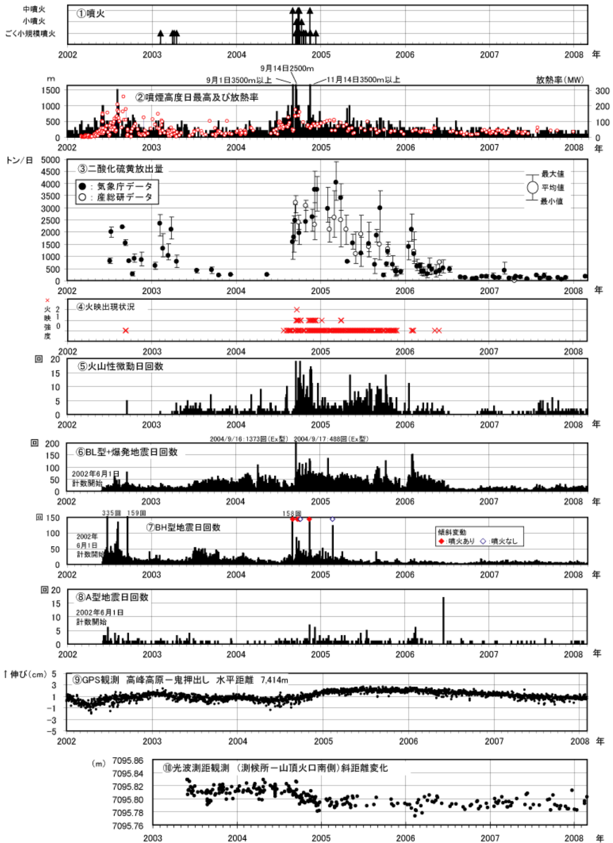
図 2 浅間山 最近の火山活動の推移（2002 年 1 月～2008 年 2 月）
