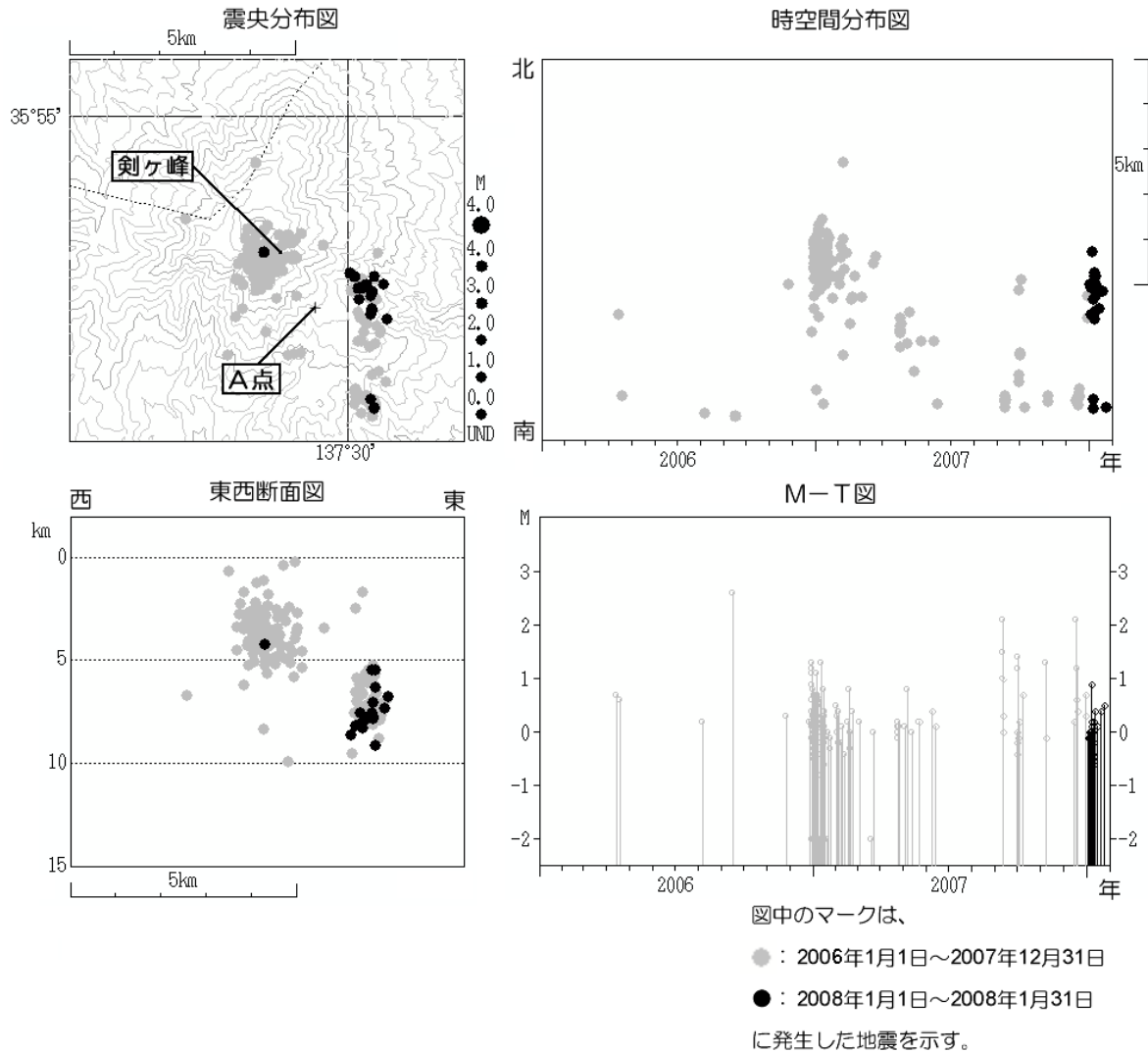
図3※ 御嶽山 山頂付近の地震活動（2006 年 1 月 1 日～2008 年 1 月 31 日） +印は気象庁地震観測点（A点）の位置を示しています。M（マグニチュード）は地震の規模を表します。図中の震源要素は一部暫定値で、後日変更することがあります。
