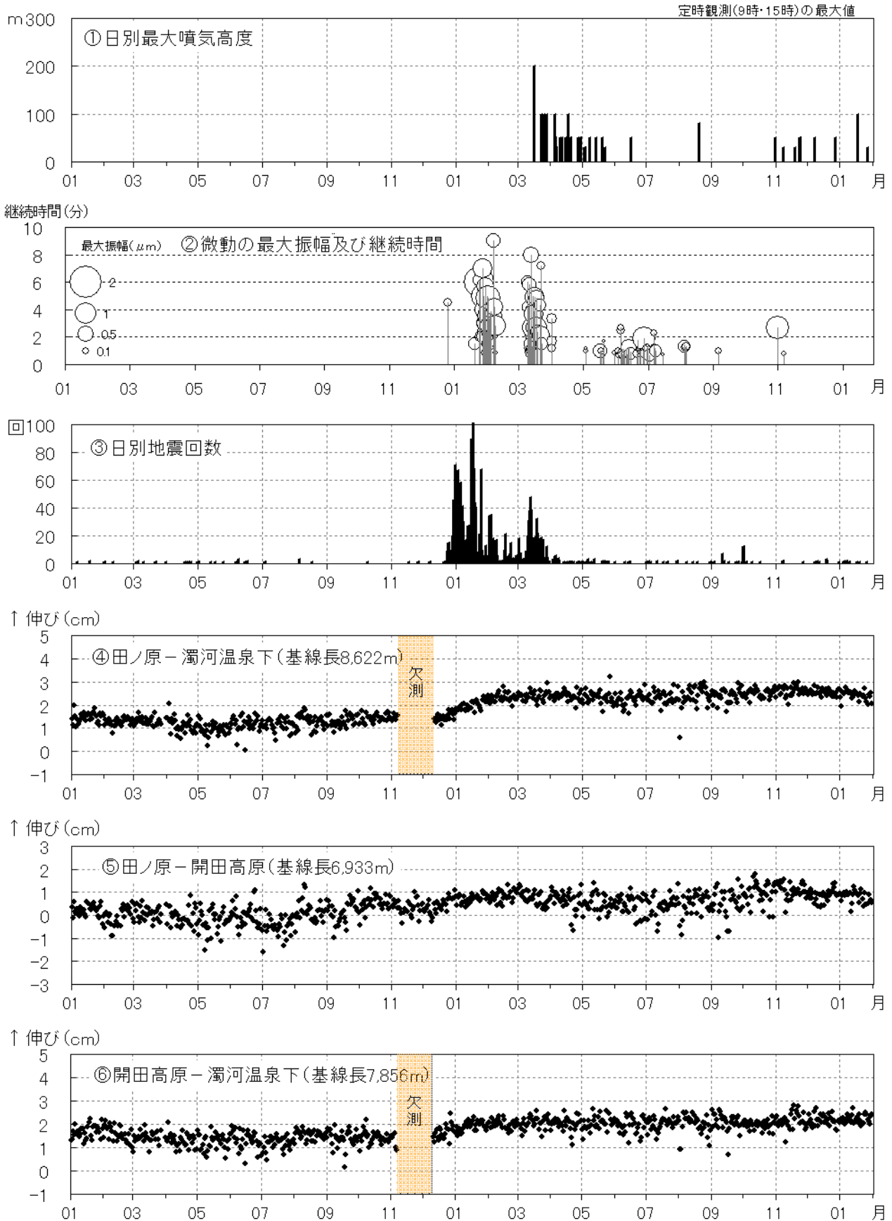
図2 御嶽山 最近の火山活動の推移 (2006 年 1 月 1 日～2008 年 1 月 31 日)
