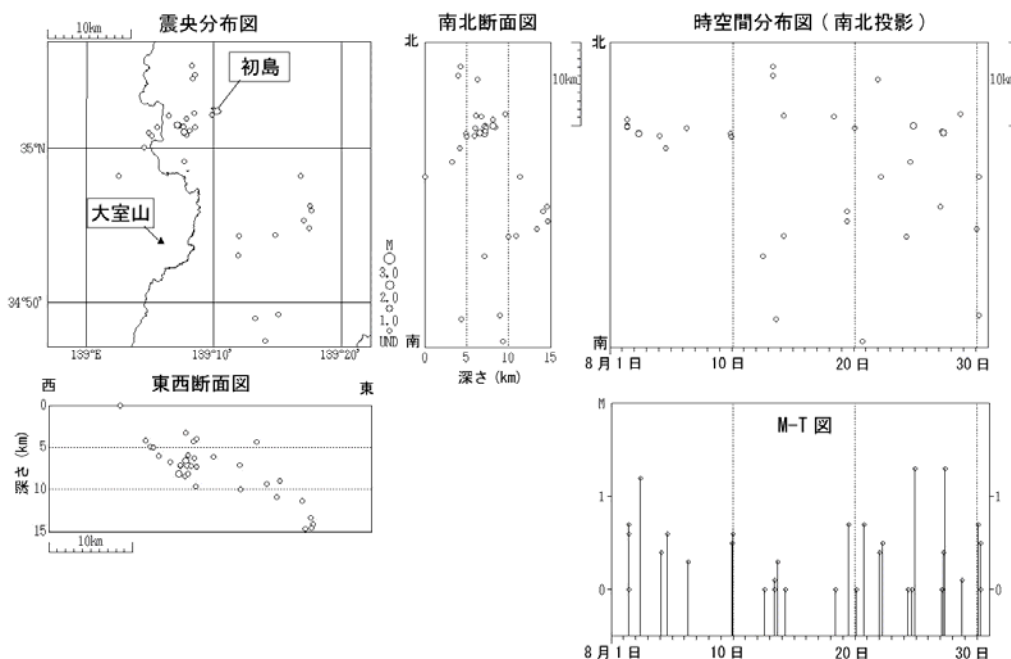
図1※ 伊豆東部火山群 地震活動経過図（2007年8月1日～8月31日）
