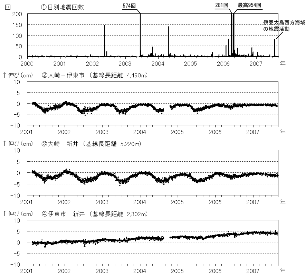
図 2 伊豆東部火山群 最近の火山活動の推移 (2001 年 1 月～2007 年 8 月)
