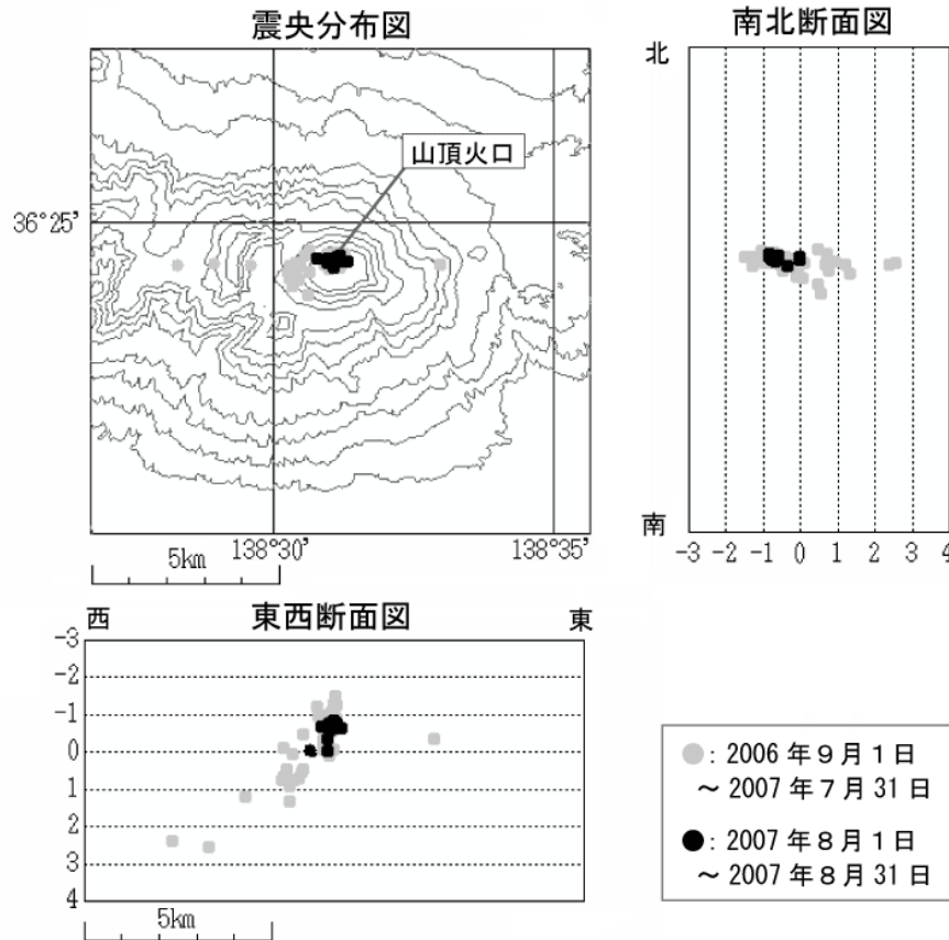
図3 浅間山 火山性地震の震源分布（2006年9月1日～2007年8月31日）
