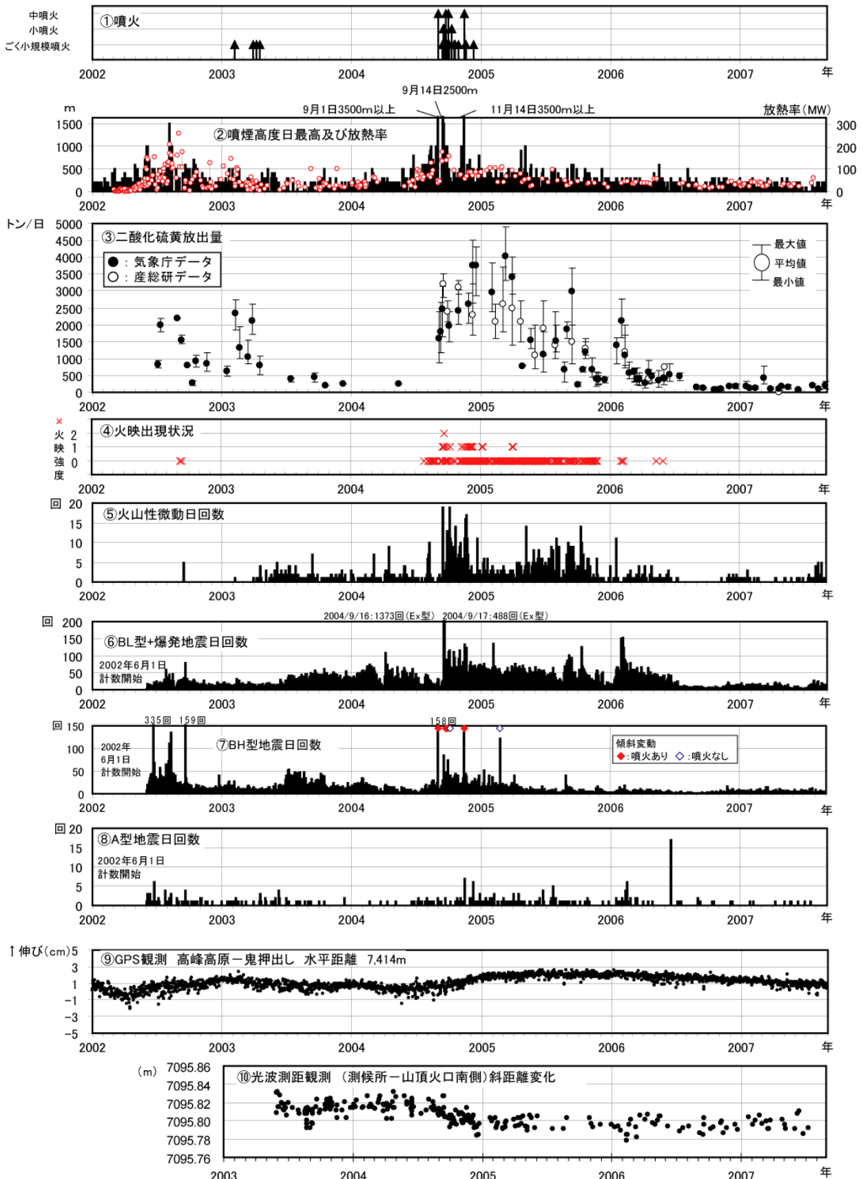
図 2 浅間山 最近の火山活動の推移（2002 年 1 月～2007 年 8 月） 産業技術総合研究所による観測結果（産総研データ）が含まれています。 脚注 4）を参照。 地震の種類別（図 5 参照）に計数を開始した 2002 年 6 月 1 日からのデータを掲載。
