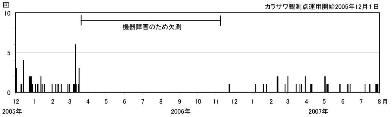
図2 新潟焼山 日別地震回数（2005年12月1日～2007年7月31日）
