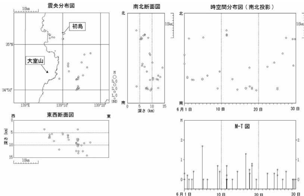
図1 伊豆東部火山群 地震活動経過図(2007年6月1日～6月30日)
