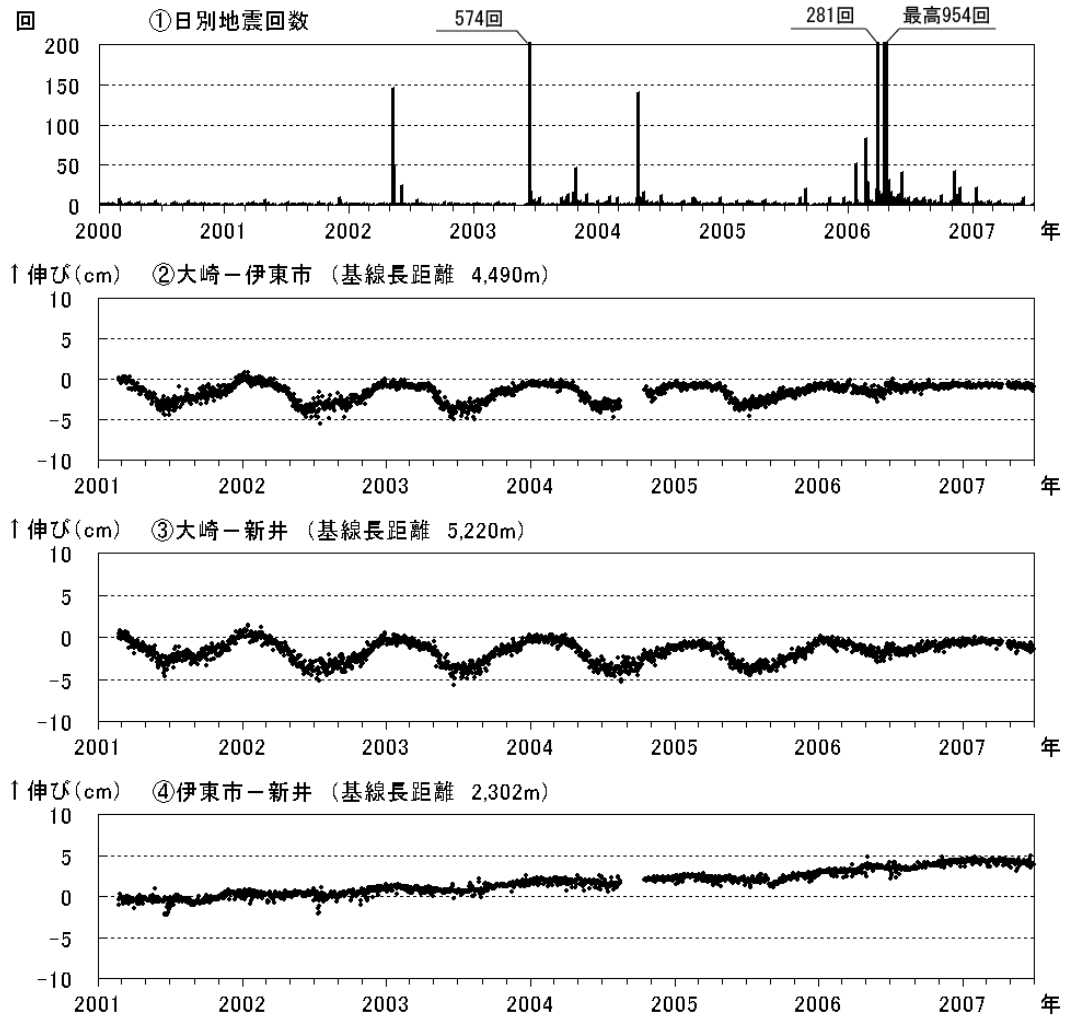
図2 伊豆東部火山群 最近の火山活動の推移（2001年1月～2007年6月）
