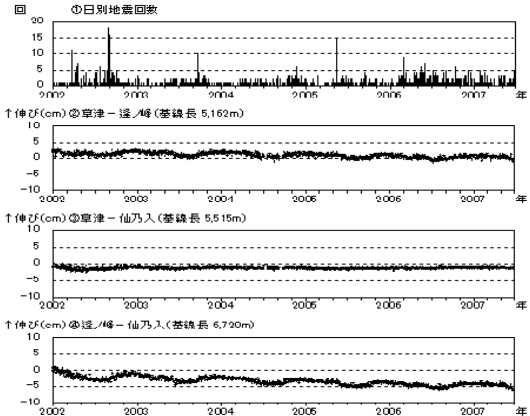
図3 草津白根山 最近の火山活動の推移(2002年1月~2007年6月)
