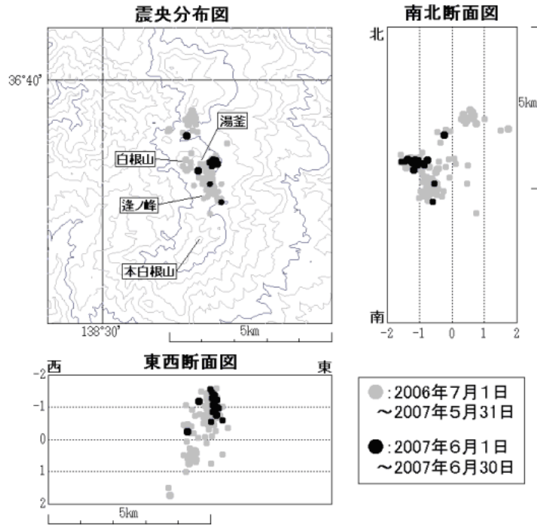
図2 草津白根山 火山性地震の震源分布(2006年7月1日~2007年6月30日)
