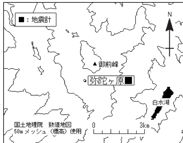
図 3 白山 気象庁の観測点配置図（小さな白丸は観測点位置を示しています）
