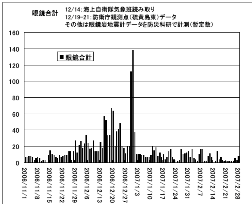
図 2 ※ 硫黄島 最近の火山性地震回数の経過（2006 年 11 月 1 日～2007 年 2 月 28 日）
