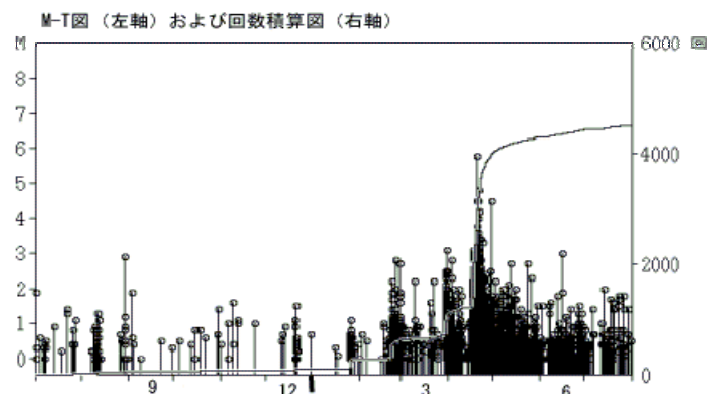
図 2 最近約 1 年間の地震活動経過
