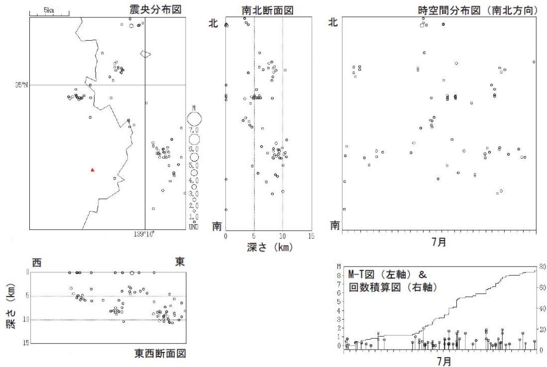
図 1 ※ 7 月の地震活動経過（2006 年 7 月 1 日～7 月 31 日、マグニチュード 1) は暫定値）
