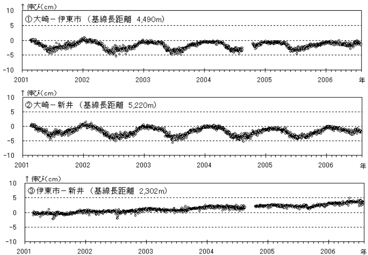
図3 伊豆東部火山群 GPS連続観測による基線長変化（2001年2月～2006年7月）
