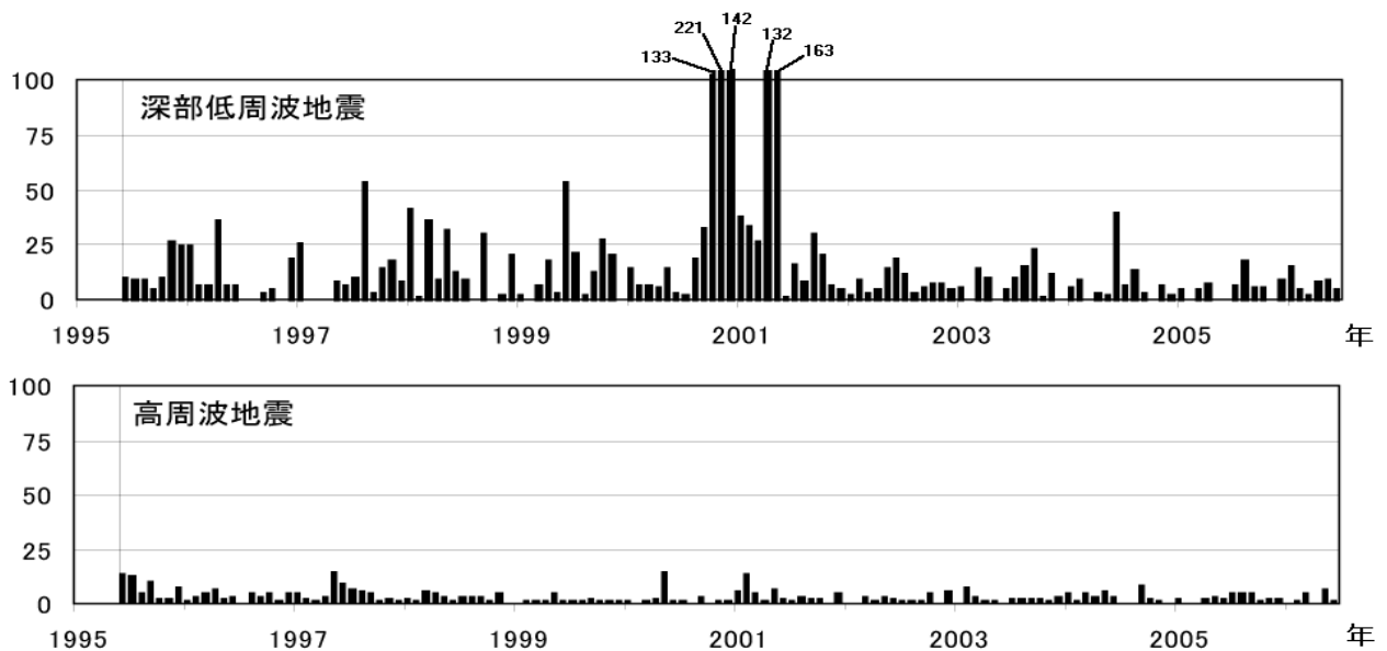
図1※ 富士山 月別地震回数（1995年6月～2006年6月）
