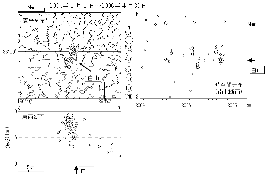
図 1 白山 広域ネットによる白山周辺の地震活動
