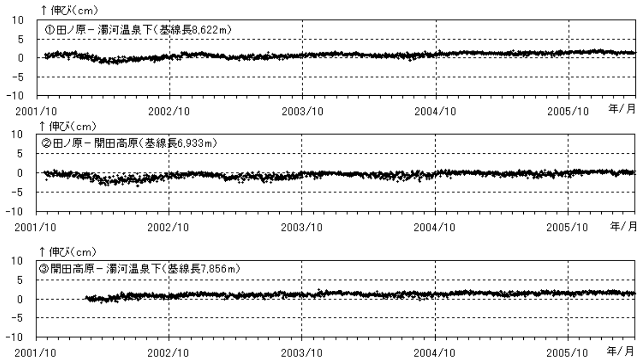
図 2 御嶽山 G P S 連続観測による基線長変化（2001 年 10 月 23 日～2006 年 4 月 30 日）
