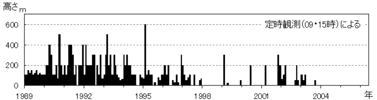
図 3 御嶽山 月別最大噴煙高度（1989年 1 月～2006年 4 月）
