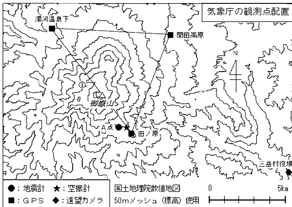
図 4 御嶽山 気象庁の観測点配置
