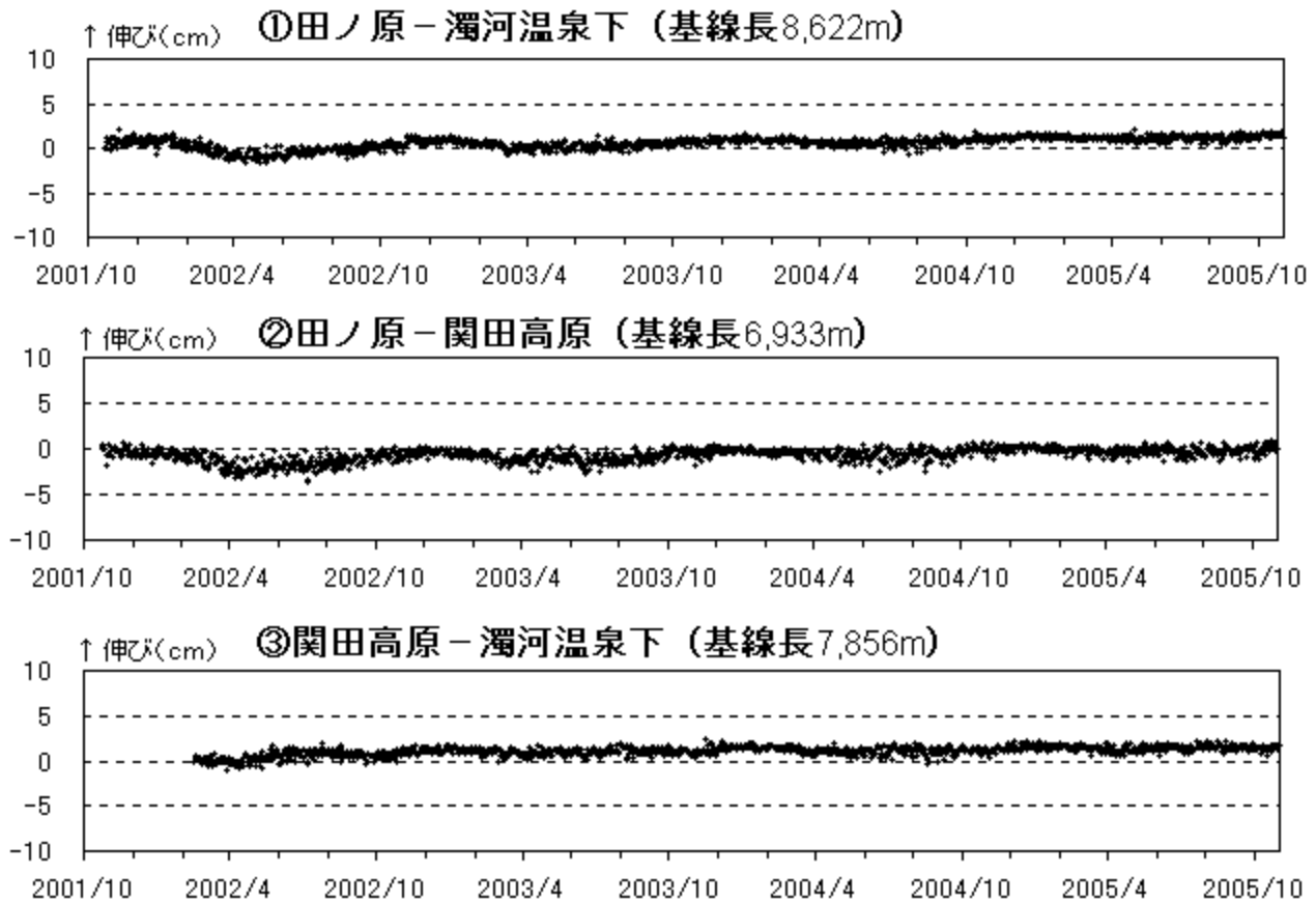
図 3 御嶽山 GPS 連続観測による基線長変化 (2001 年 10 月 23 日～2005 年 10 月 31 日)
