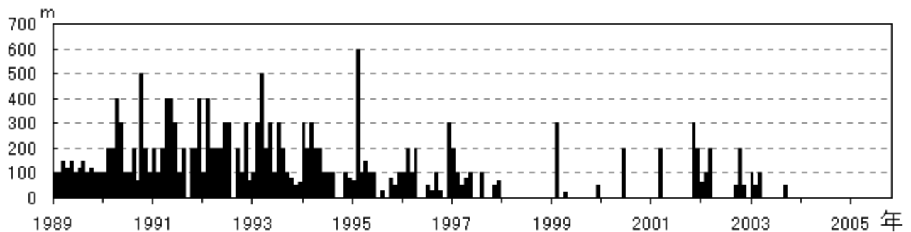
図 2 御嶽山 月別最大噴煙高度（1989 年 1 月～2005 年 10 月）
