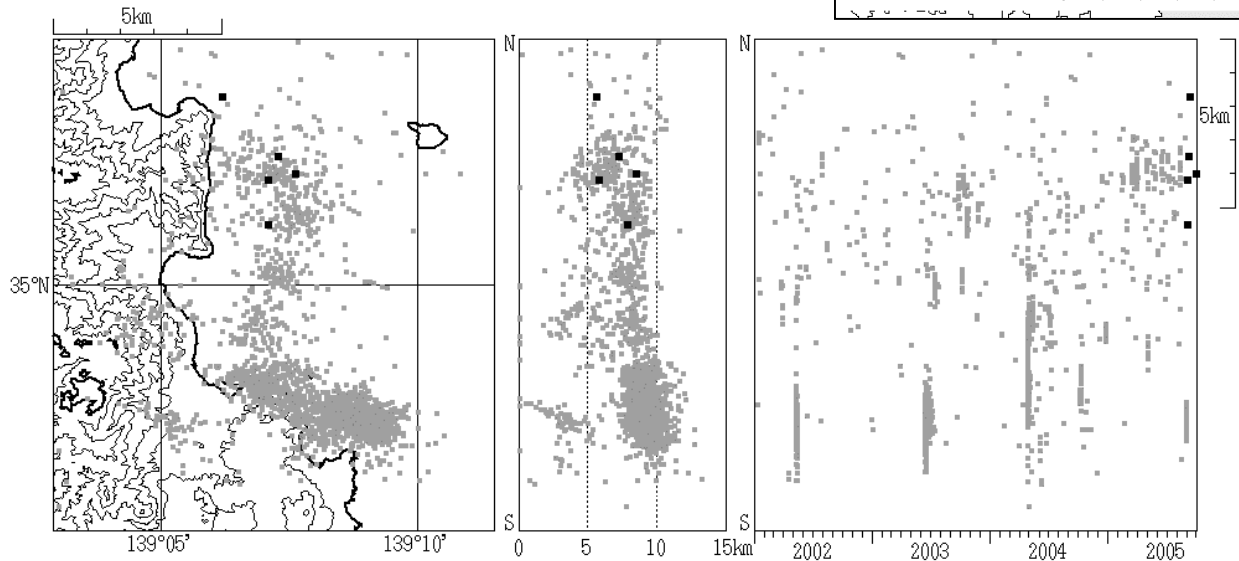
図 1 伊豆東部火山群 震源分布図
