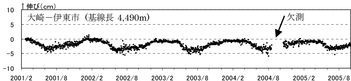
図 2 伊豆東部火山群 GPS 連続観測による基線長変化（2001 年 2 月～2005 年 9 月）
