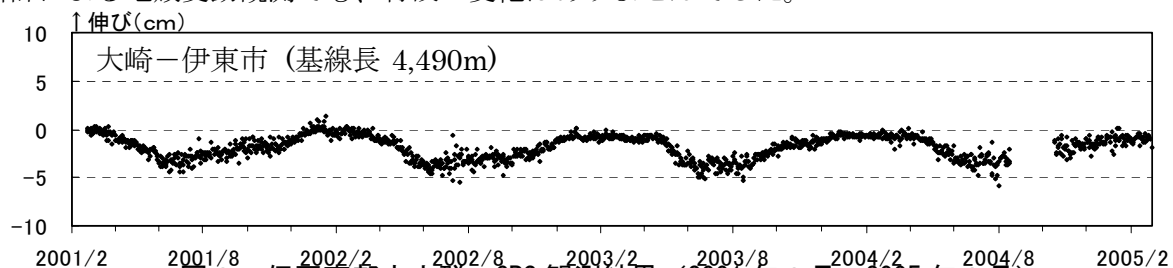
図 2 伊豆東部火山群 GPS 観測結果（2001 年 2 月～2005 年 2 月）
