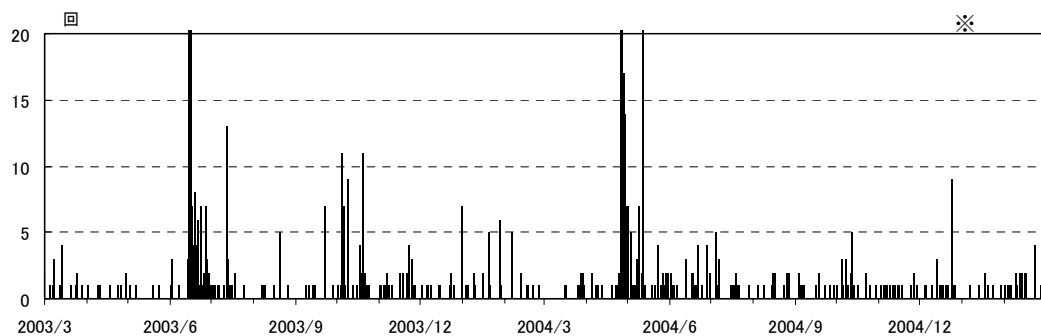
図 1 伊豆東部火山群 火山性地震日別回数（2003 年 3 月 1 日～2005 年 2 月 28 日）
