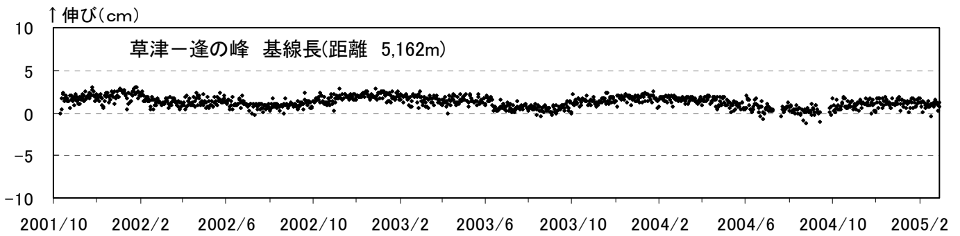
図2 草津白根山 GPS観測結果(基線長変化) (2001年10月1日～2005年2月28日) その他の基線でも火山活動によるとみられる変化は観測されていない。
