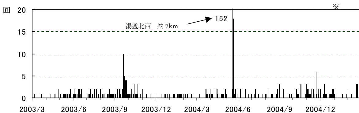
図1 草津白根山 火山性地震日別回数（2003年3月1日～2005年2月28日）
