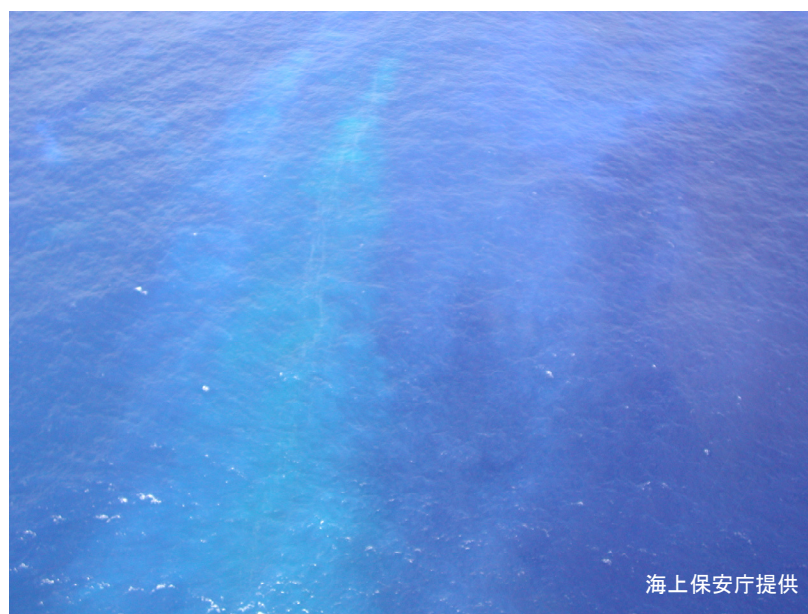
図1 福德岡ノ場 変色水の様子（2004年10月13日）
