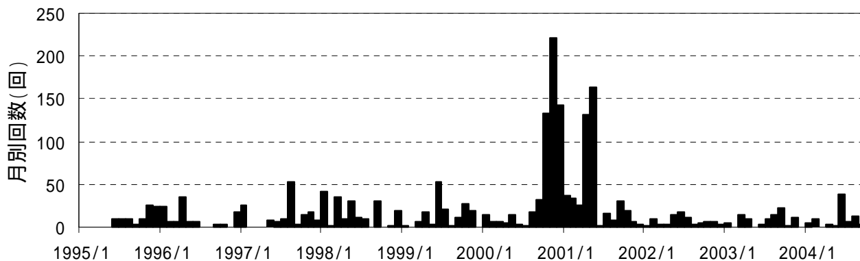
図2 富士山 低周波地震月別回数(1995年6月～2004年9月)
