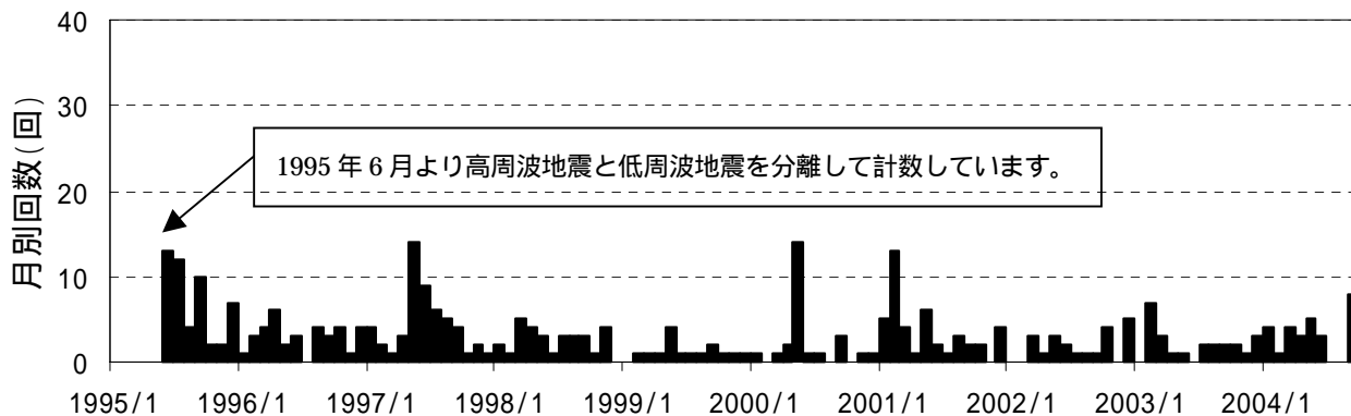
図1 富士山 高周波地震月別回数(1995年6月～2004年9月)
