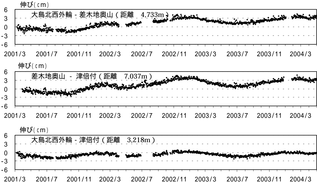
図2 伊豆大島 GPS 観測結果(基線長変化) (2001 年 3 月 7 日 ~ 2004 年 4 月 30 日) 火口を挟む と の基線では年周変動以外に長期的な伸びの傾向が見られる
