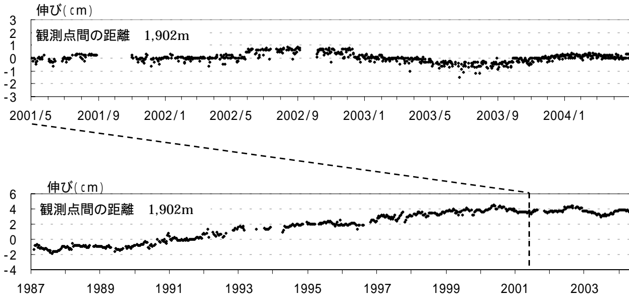
図3 伊豆大島 光波距離計 (津倍付 - 神達) 斜距離変化日平均値 (1987 年 ~ 2004 年) 上: 日平均値 (2001 年 3 月 1 日 ~ 2004 年 4 月 30 日) 下: 旬平均値 (1987 年 1 月 ~ 2004 年 4 月)
