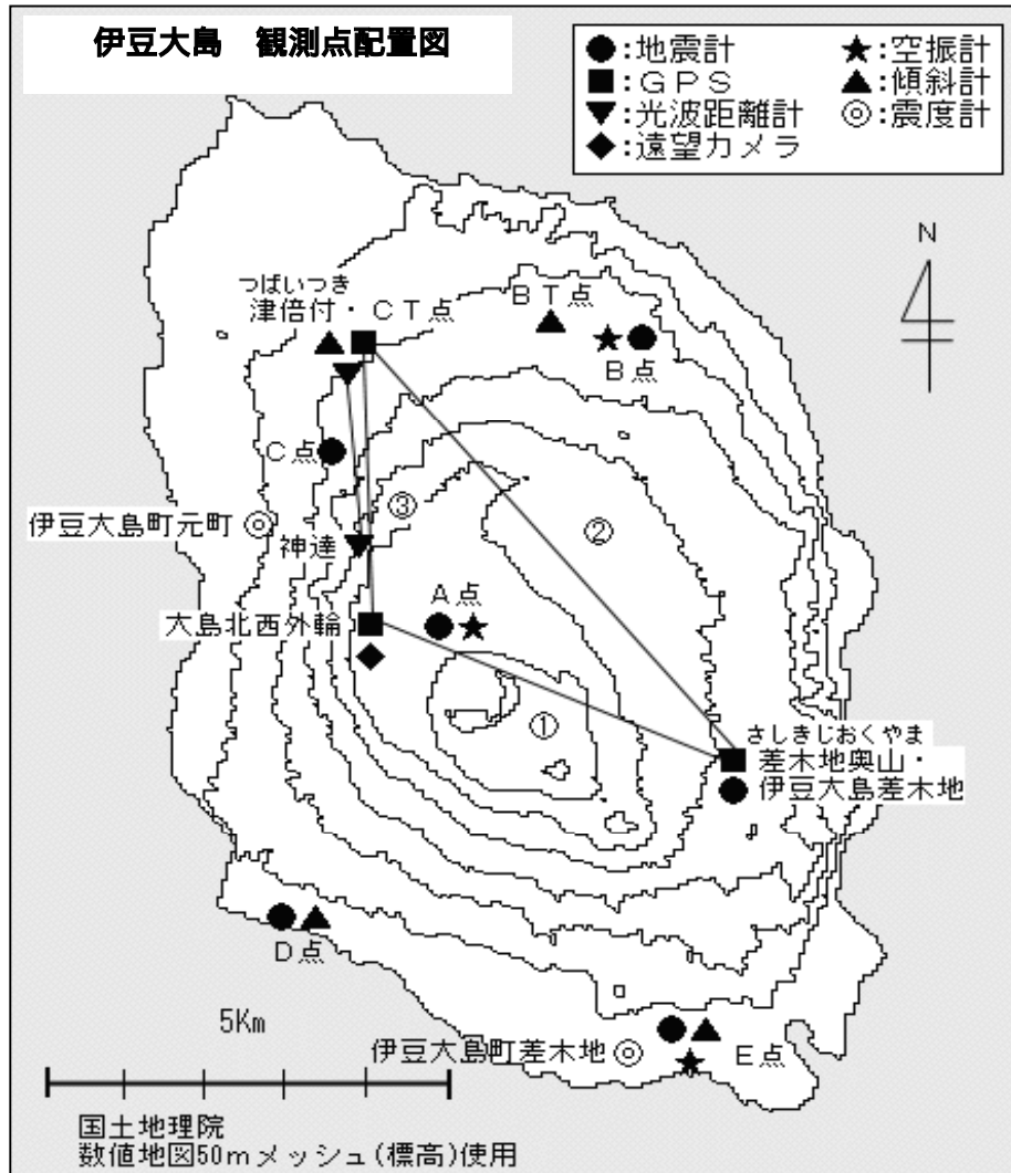
図4 伊豆大島 気象庁の観測点配置
