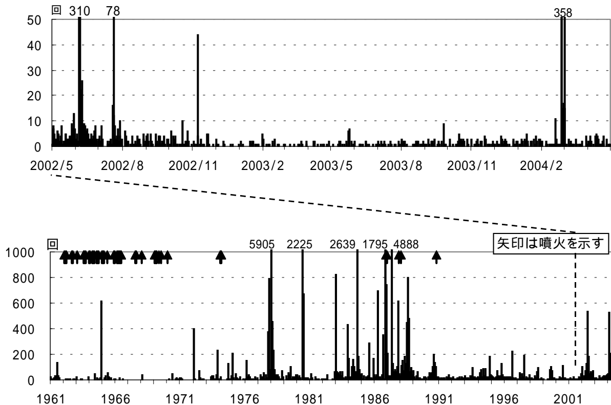
図1 伊豆大島 火山性地震回数 (1961 年 1 月 ~ 2004 年 4 月)
