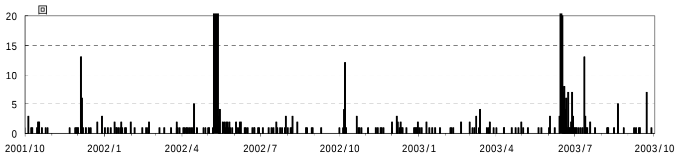
図 1 伊豆東部火山群 火山性地震日別回数（2001 年 10 月 1 日～2003 年 9 月 30 日）
