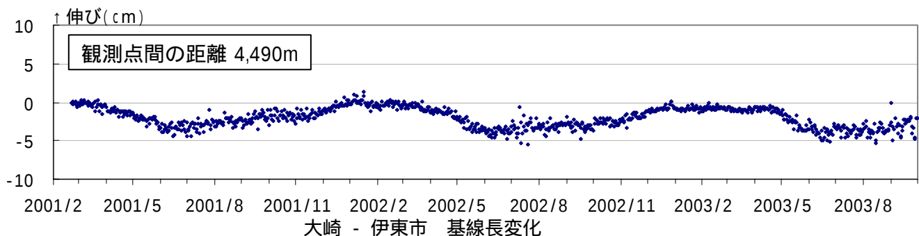
図 2 伊豆東部火山群 GPS 観測結果（2001 年 2 月 1 日～2003 年 9 月 30 日）
