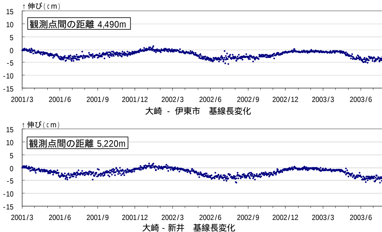
図 3 伊豆東部火山群 GPS 観測結果（2001 年 3 月 1 日～2003 年 7 月 31 日）
