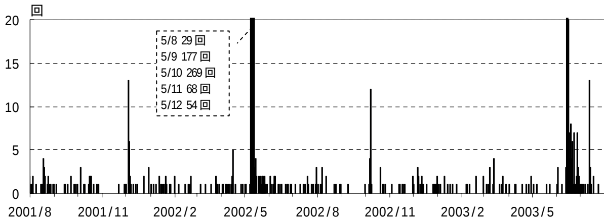
図 1 伊豆東部火山群 火山性地震日別回数（2001 年 8 月 1 日～2003 年 7 月 31 日）
