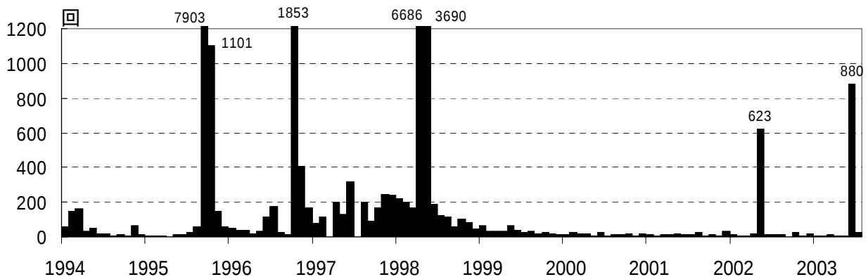
図 2 伊豆東部火山群 火山性地震月別回数（1994 年 1 月～2003 年 7 月）
