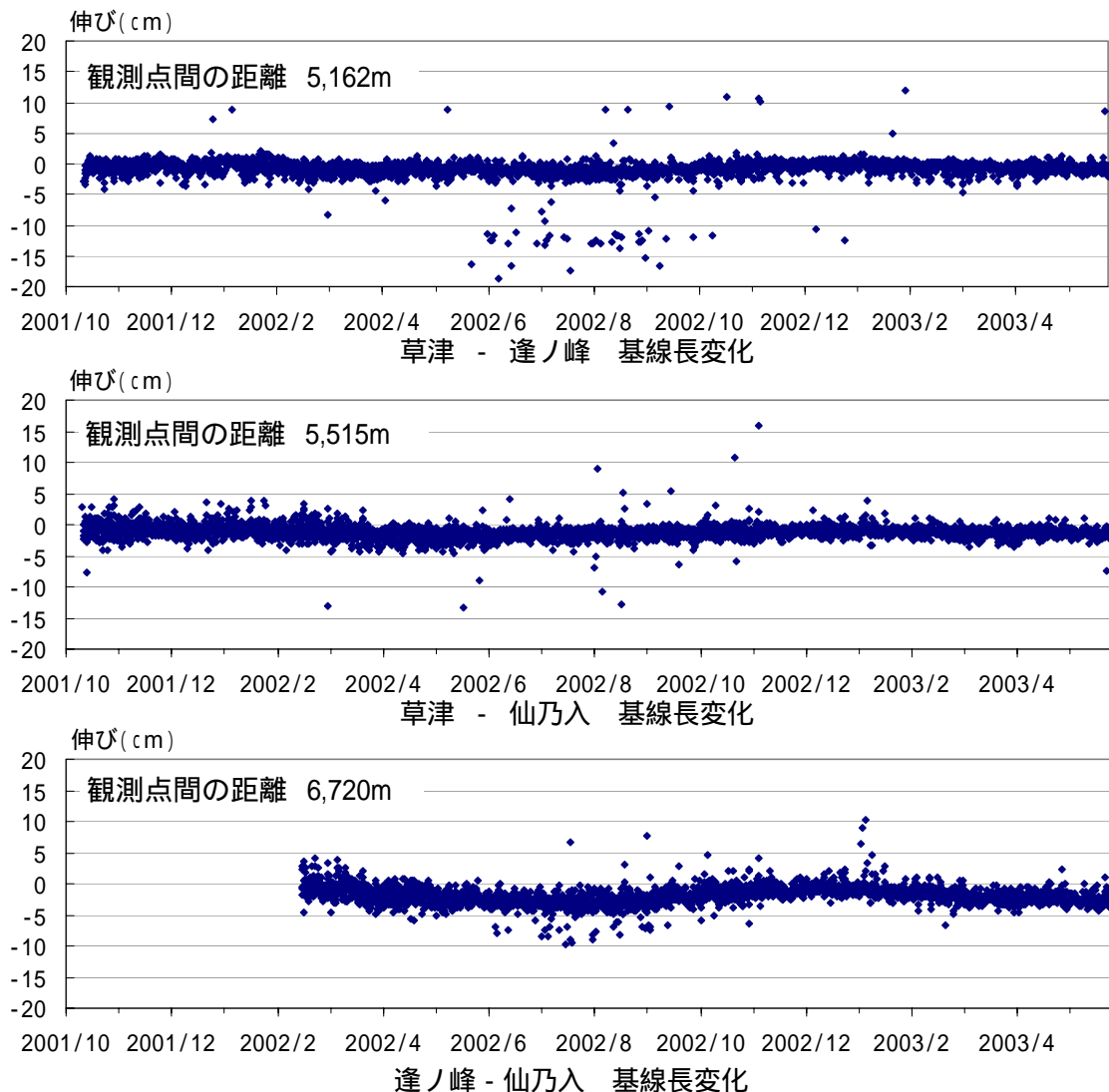
図3 草津白根山 GPS観測結果(2001年10月1日~2003年5月31日)
