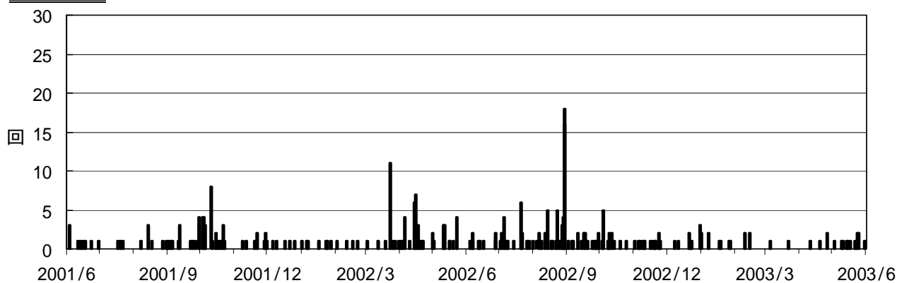
図1 草津白根山 火山性地震日別回数(2001年6月1日~2003年5月31日)
