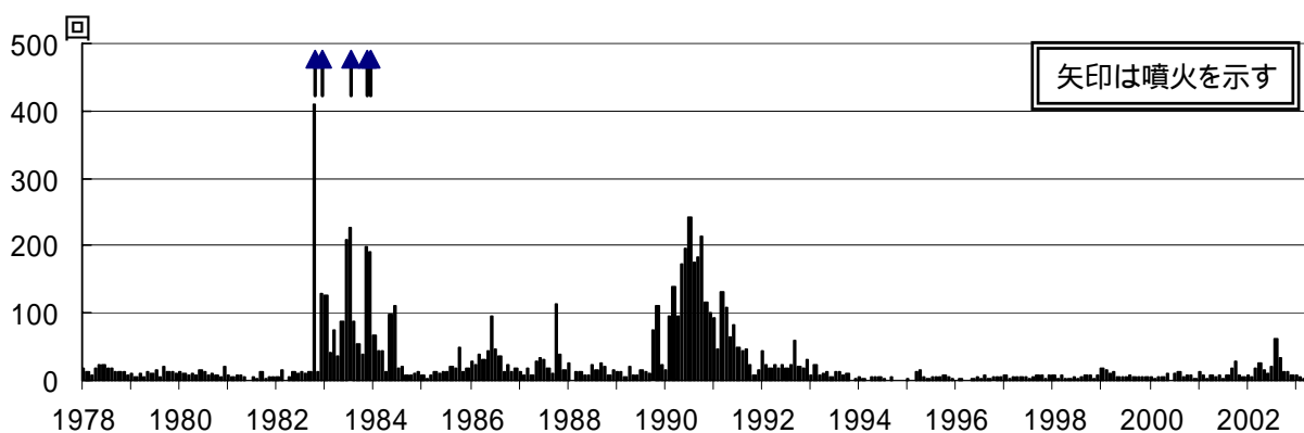
図2 草津白根山 火山性地震月別回数及び噴火状況(1978年1月~2003年5月)
