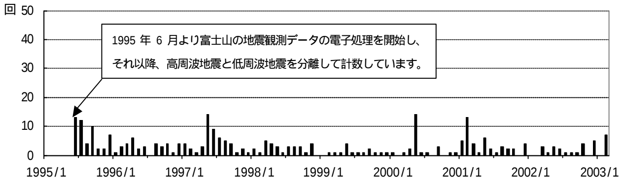
図 3 富士山 高周波地震月別回数 (1995 年 6 月 ~ 2003 年 2 月)
