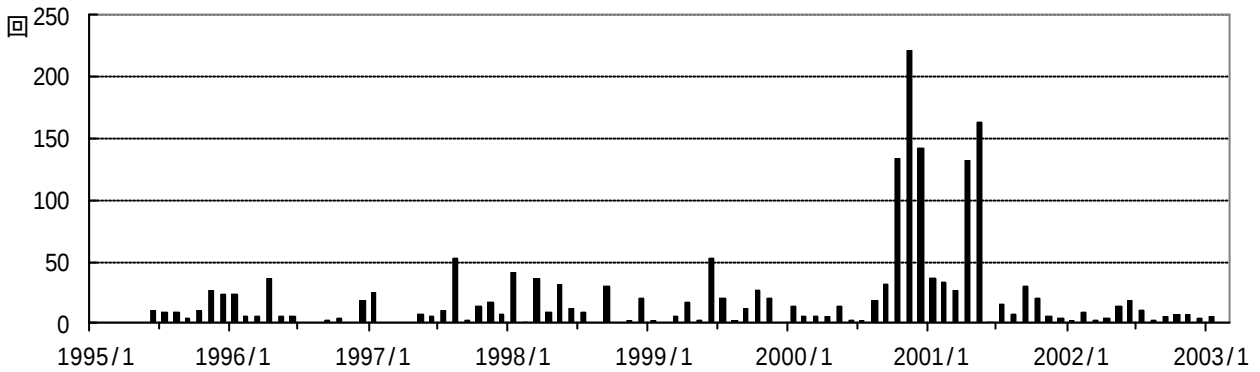
図 4 富士山 低周波地震月別回数 (1995 年 6 月 ~ 2003 年 2 月)
