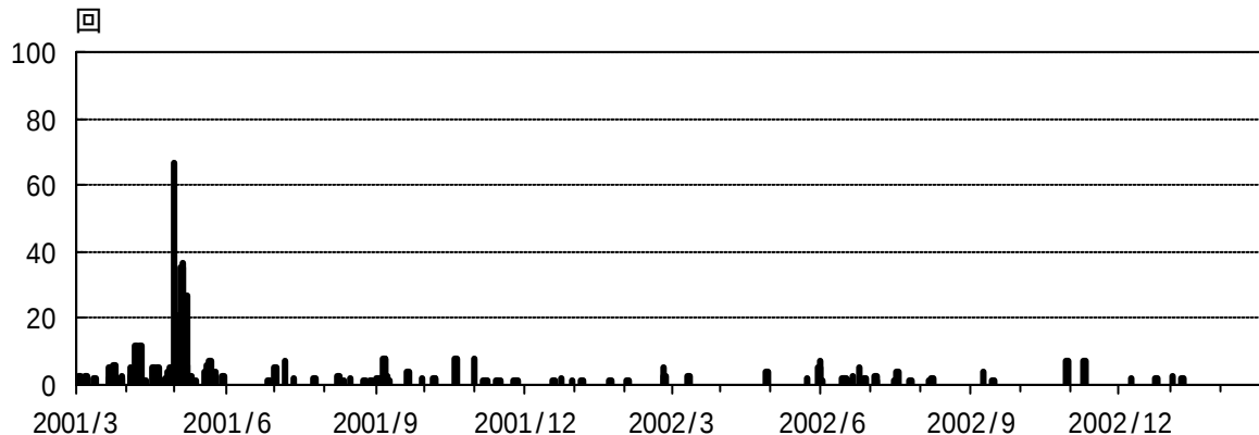
図 2 富士山 低周波地震日別回数（2001年3月 1日～2003年2月28日）
