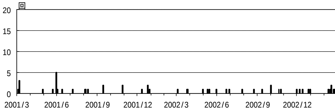
図 1 富士山 高周波地震日別回数（2001年3月 1日～2003年2月28日）
