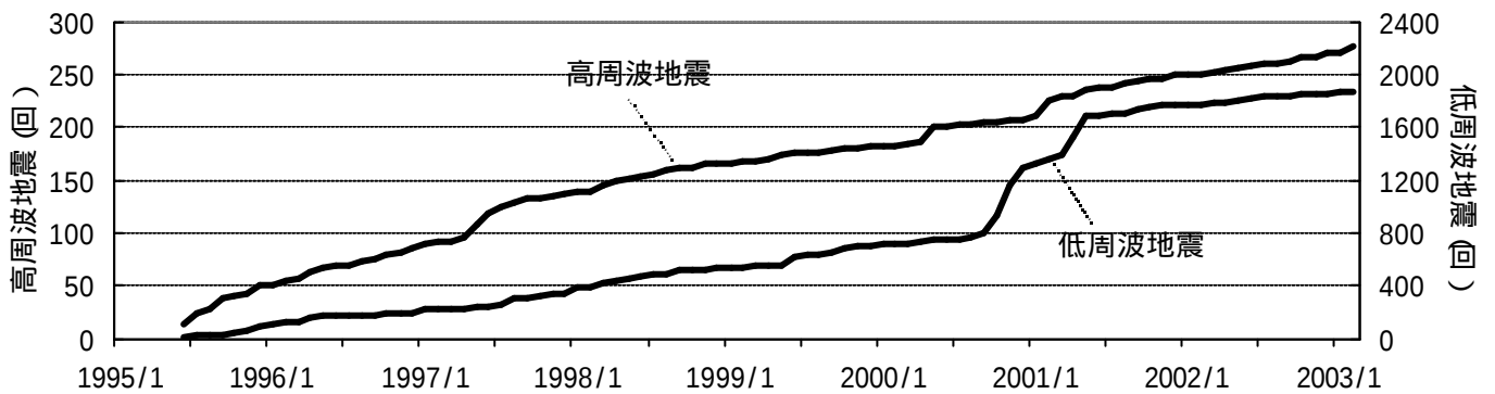
図 5 富士山 地震積算回数 (1995 年 6 月 ~ 2003 年 2 月)
