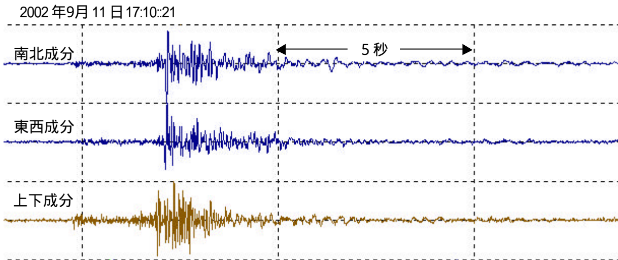
図2 日光白根山 高周波地震波形例
