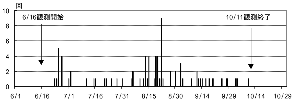
図1 日光白根山 火山性地震日別回数(2002年6月16日～10月11日)
