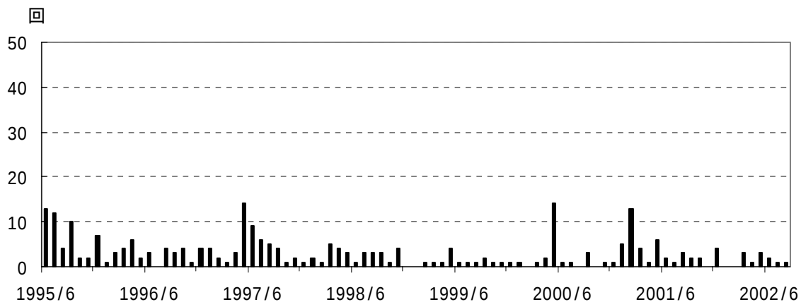
図3 富士山 高周波地震月別回数(1995年6月～2002年8月)
