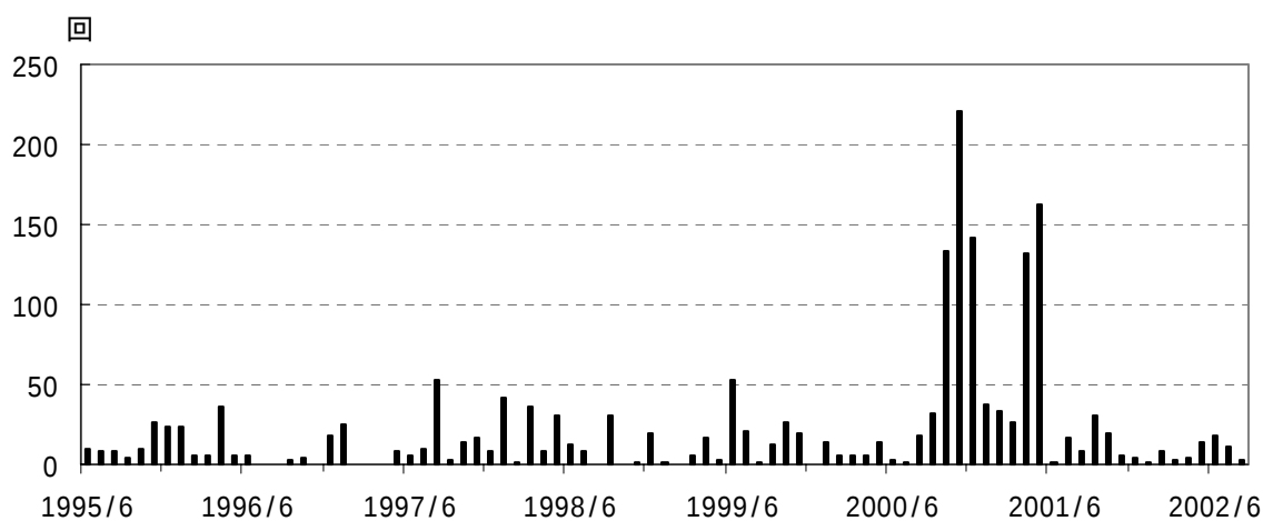
図4 富士山 低周波地震月別回数(1995年6月～2002年8月)
