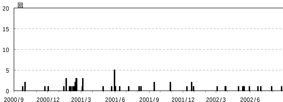
回 図1 富士山 高周波地震日別回数(2000年9月1日～2002年8月31日)
