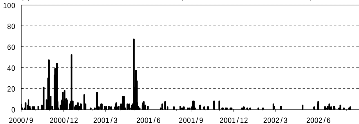
回 図2 富士山 低周波地震日別回数(2000年9月1日～2002年8月31日)
