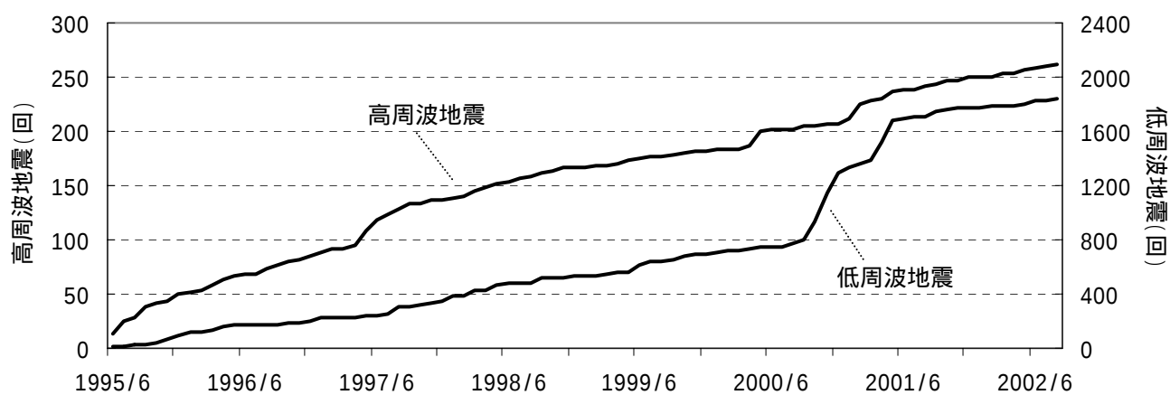
図5 富士山 地震積算回数(1995年6月～2002年8月)
