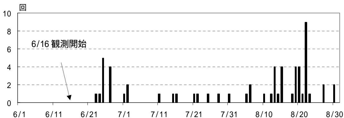
図1 日光白根山 火山性地震日別回数(2002年6月16日～8月31日)
