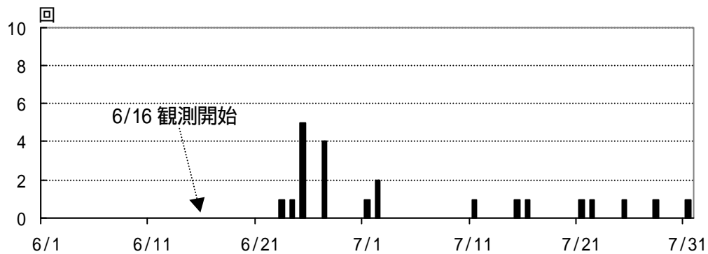
日光白根山 火山性地震日別回数(2002年 6月16日～7月31日)
