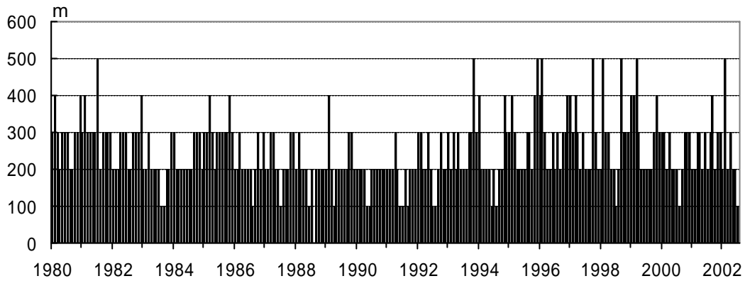
那須岳 月別最高噴煙高度 (1980年1月~2002年7月)
