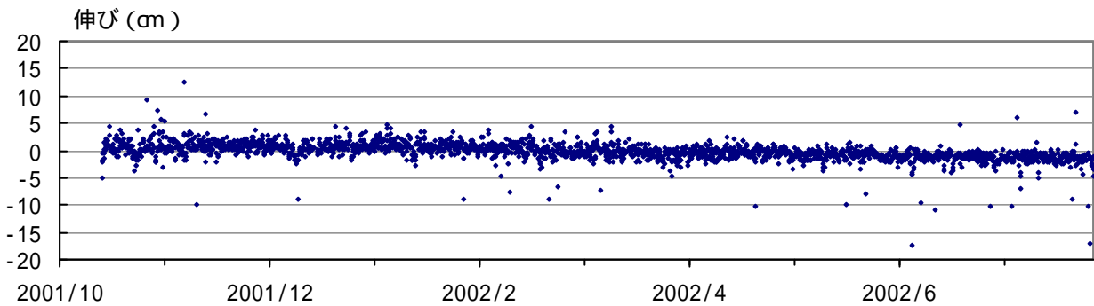
那須岳 GPS観測結果(2001年10月1日~2002年7月31日) 那須小学校 - 峠茶屋 基線長
