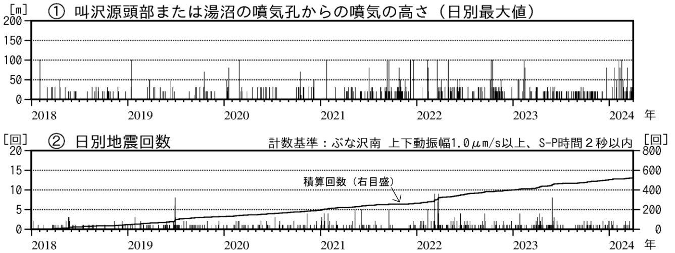
図8 秋田焼山 火山活動経過図（2018年1月～2024年3月）
