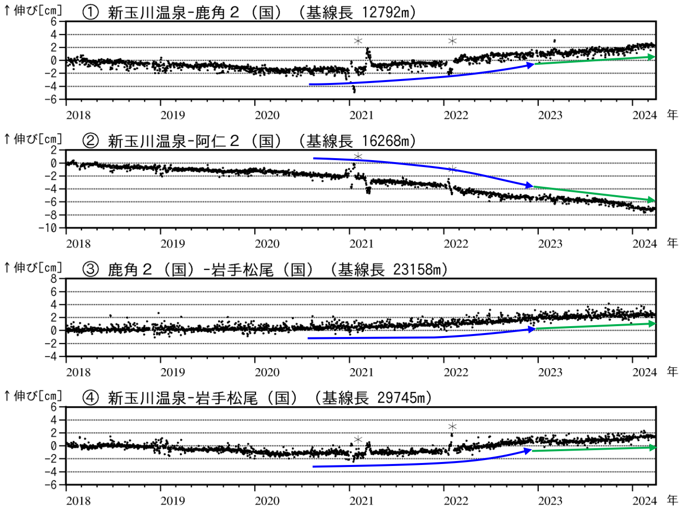
図9 秋田焼山 GNSS 基線長変化図（2018年1月～2024年3月）
