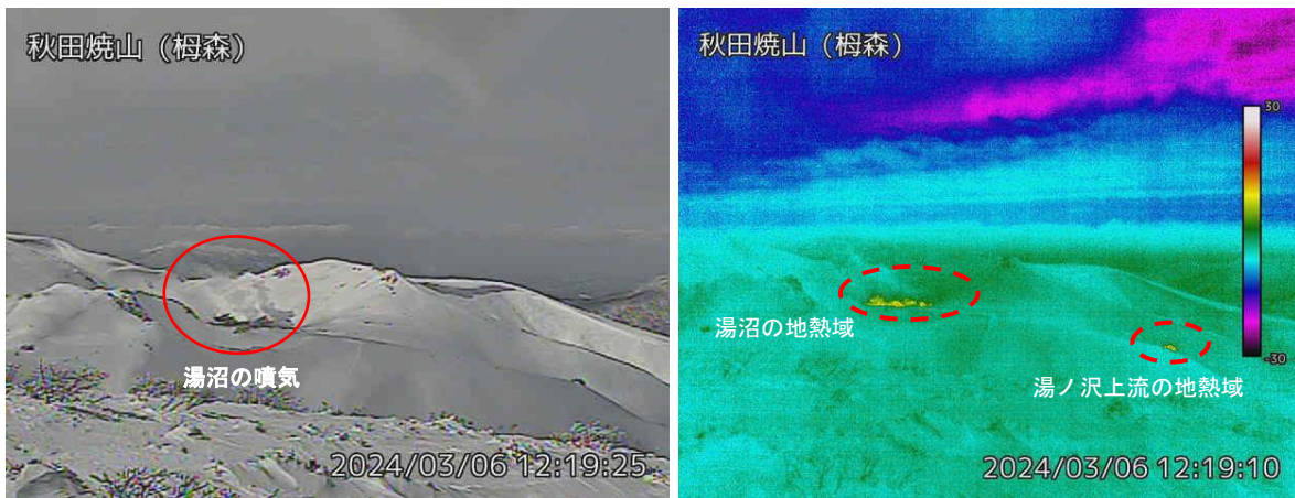
図2 秋田焼山 湯沼と湯ノ沢上流の様相と地表面温度分布（3月6日） ・柵森監視カメラ（湯沼の東約1km）の映像です。
