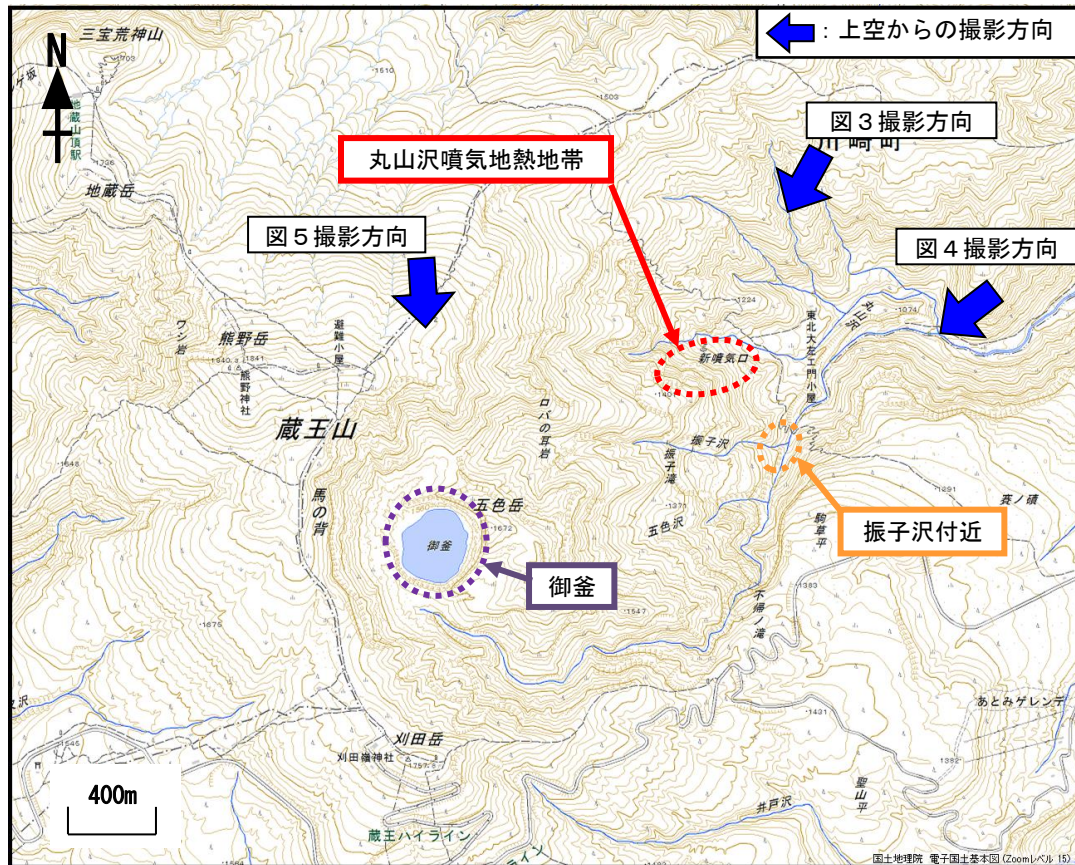
図2 蔵王山 上空から撮影した写真と地表面温度分布撮影方向
