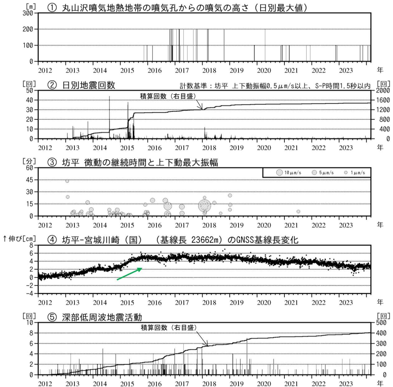
図6 蔵王山 火山活動経過図（2012年1月～2024年2月）
