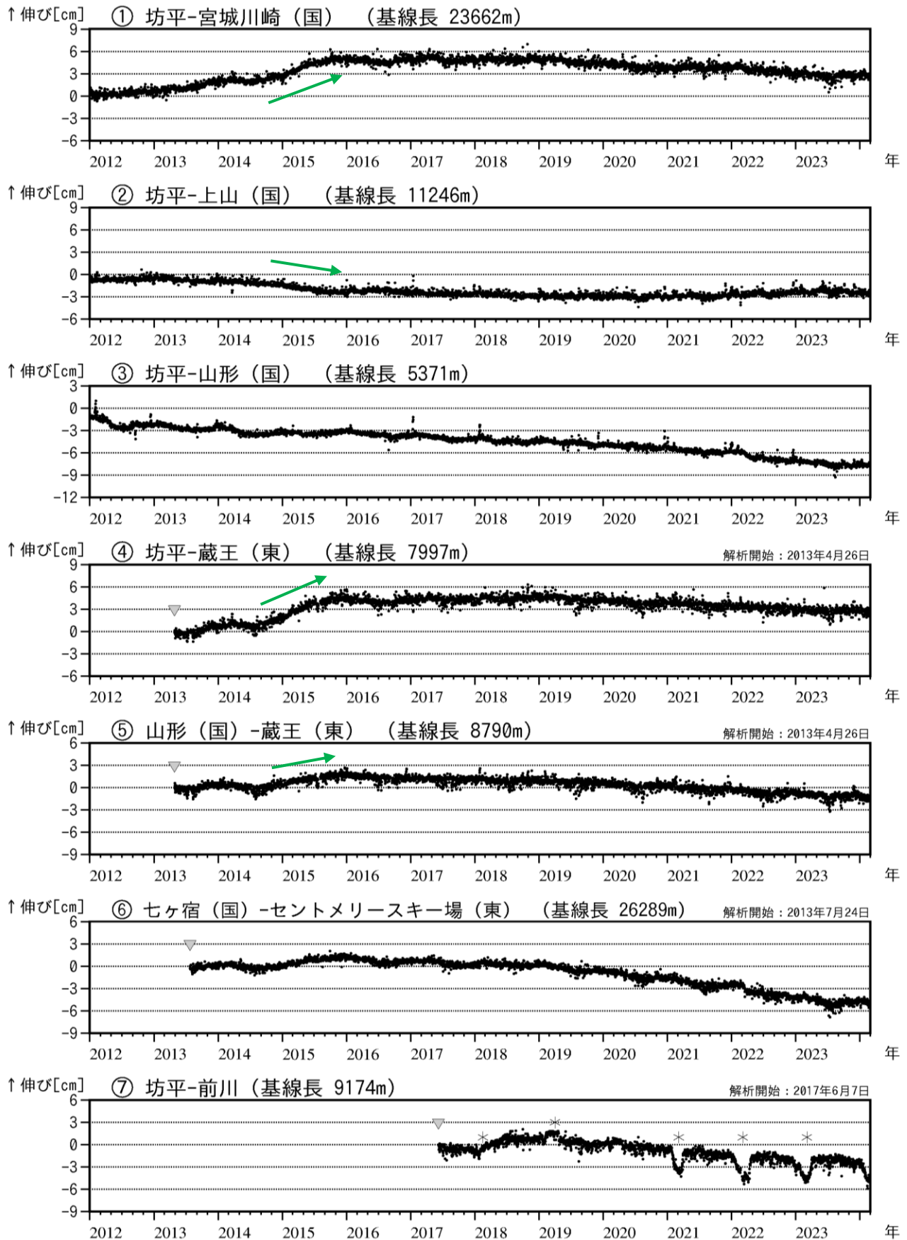
図7 蔵王山 GNSS 基線長変化図 (2012年1月～2024年2月)
