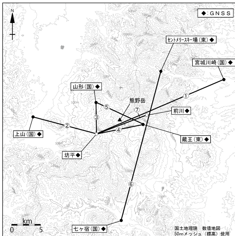
図9 蔵王山 GNSS 観測基線図
