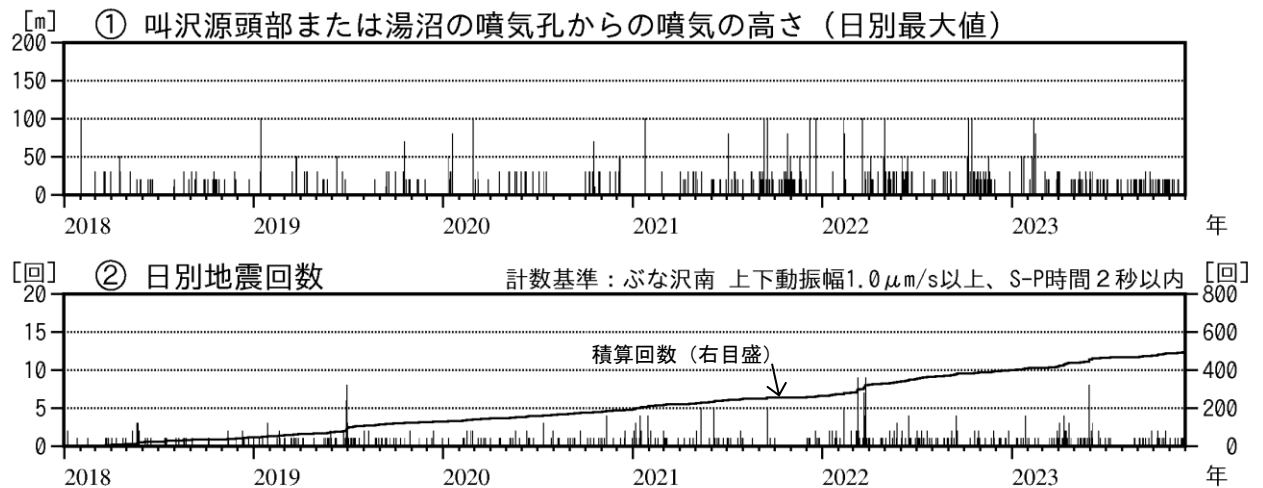
図3 秋田焼山 火山活動経過図（2018年1月～2023年11月）
