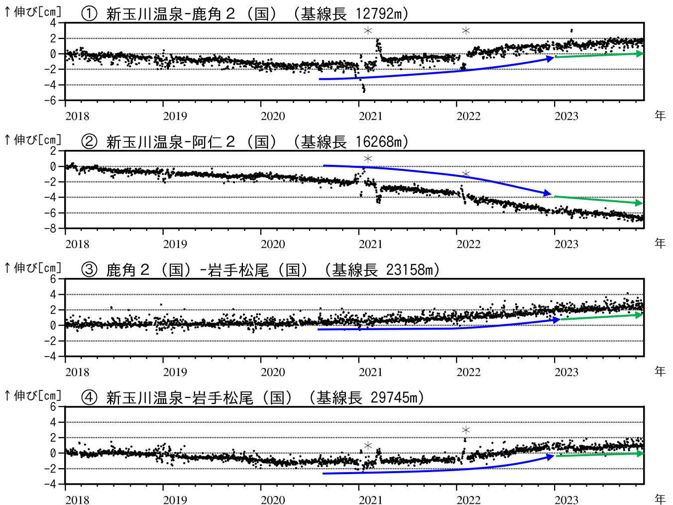
図4 秋田焼山 GNSS 基線長変化図（2018年1月～2023年11月）
