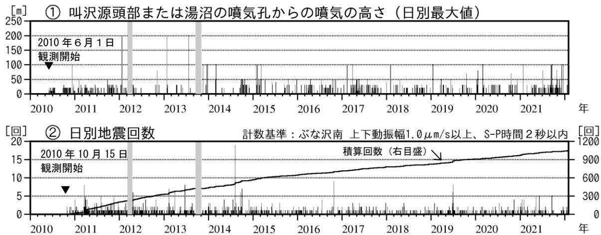
図2 秋田焼山 火山活動経過図（2010年6月～2022年1月）
