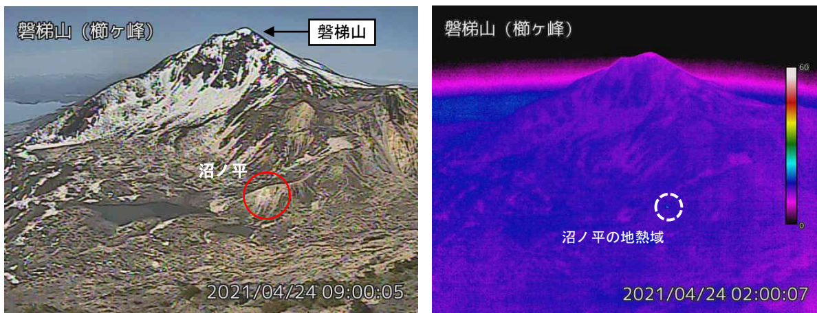
図2 磐梯山 沼ノ平周辺の状況と地表面温度分布（4月24日）
