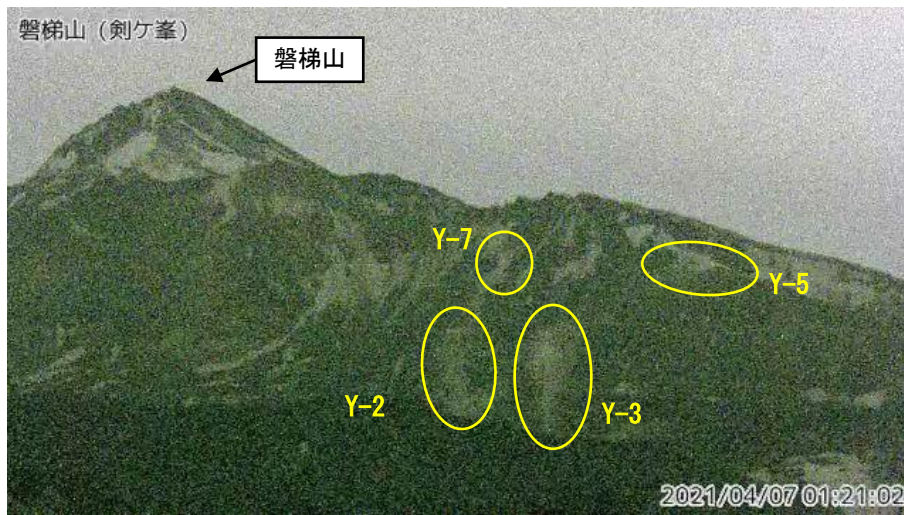
図1 磐梯山 山体北側火口壁の噴気の状態（4月7日）
