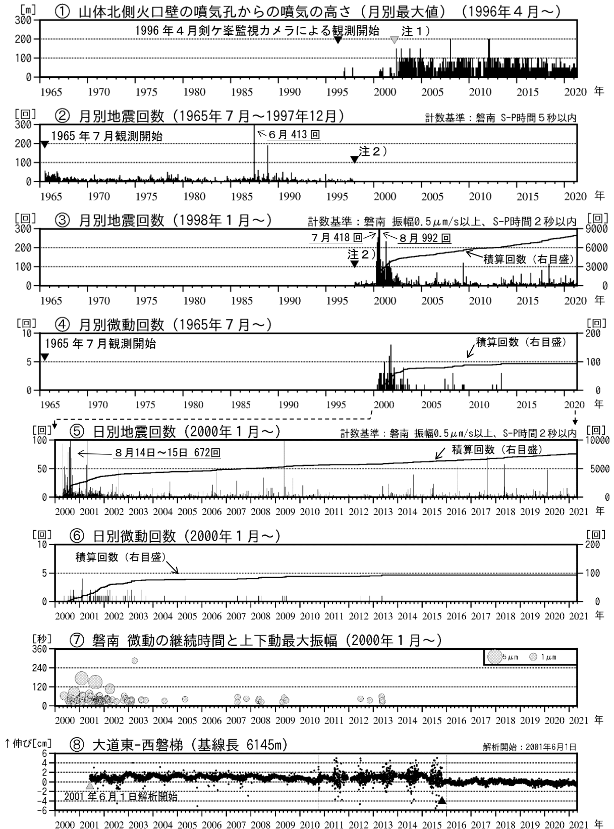
図3 磐梯山 火山活動経過図（1965年7月～2021年4月）
