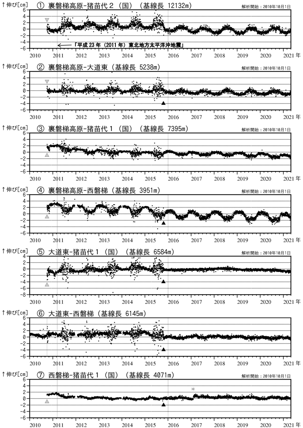
図4 磐梯山 GNSS 基線長変化図（2010年1月～2021年4月）
