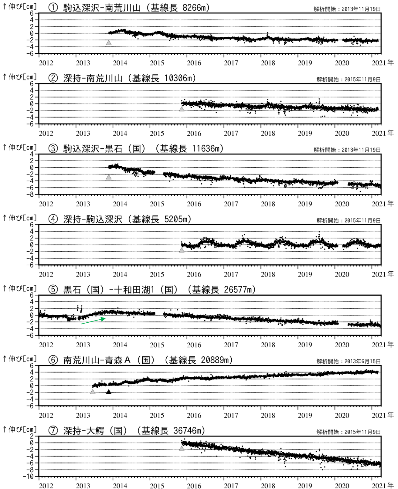
図3 八甲田山 GNSS 基線長変化図（2012年1月～2021年3月）
